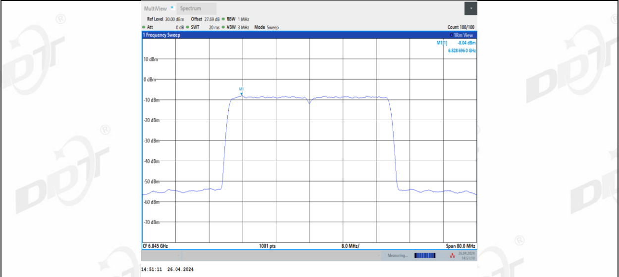
11BE40MIMO_Ant3_6845
