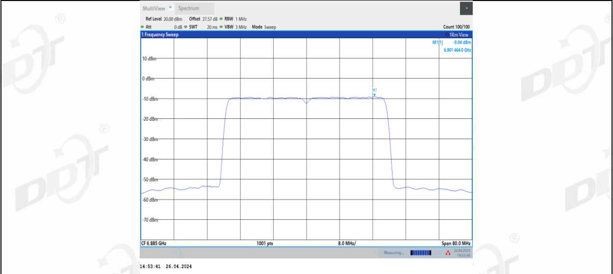
11BE40MIMO_Ant3_6885
