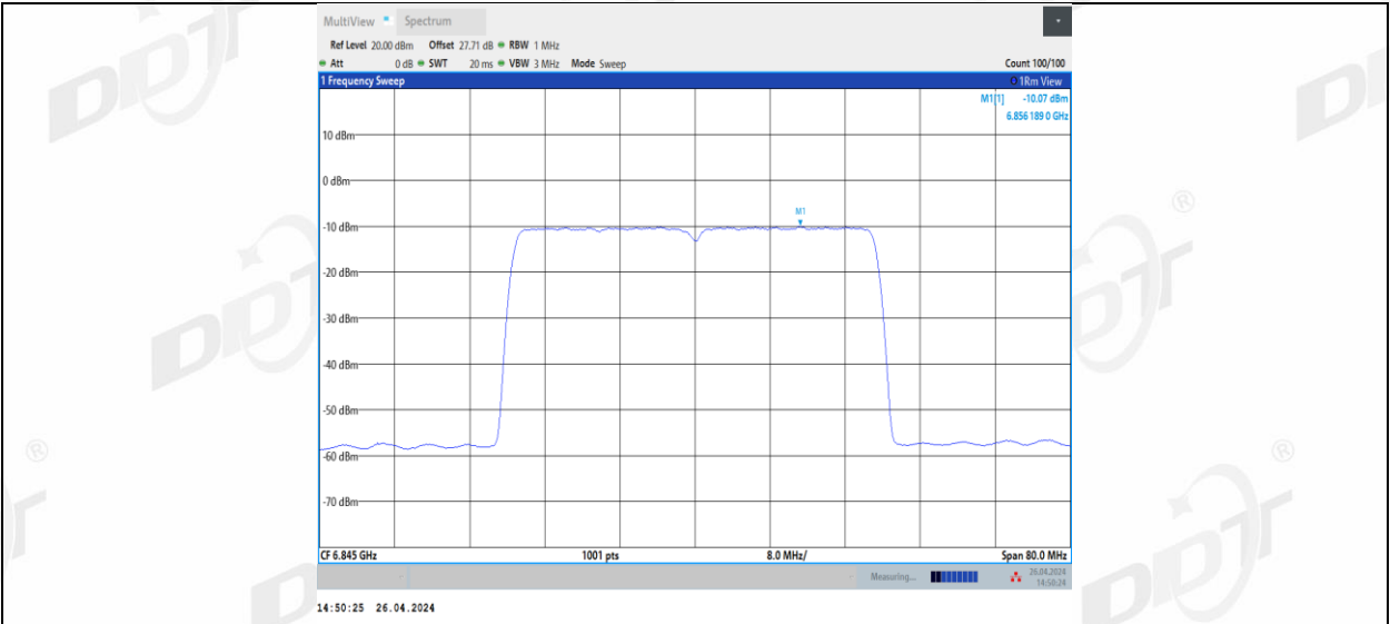
11BE40MIMO_Ant2_6845
