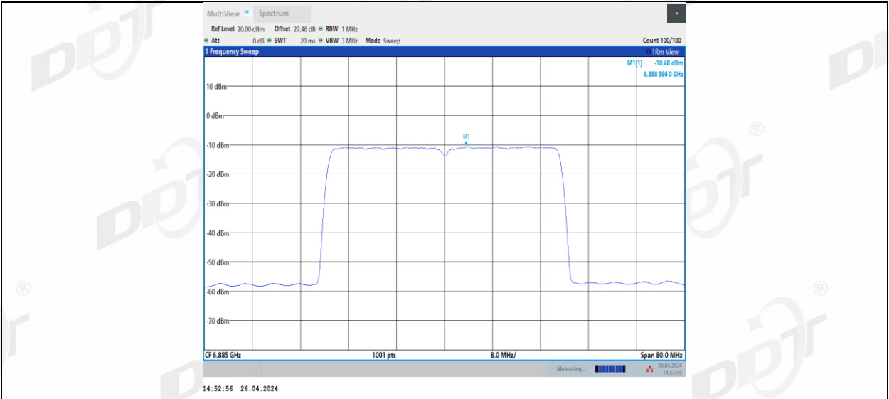
11BE40MIMO_Ant2_6885
