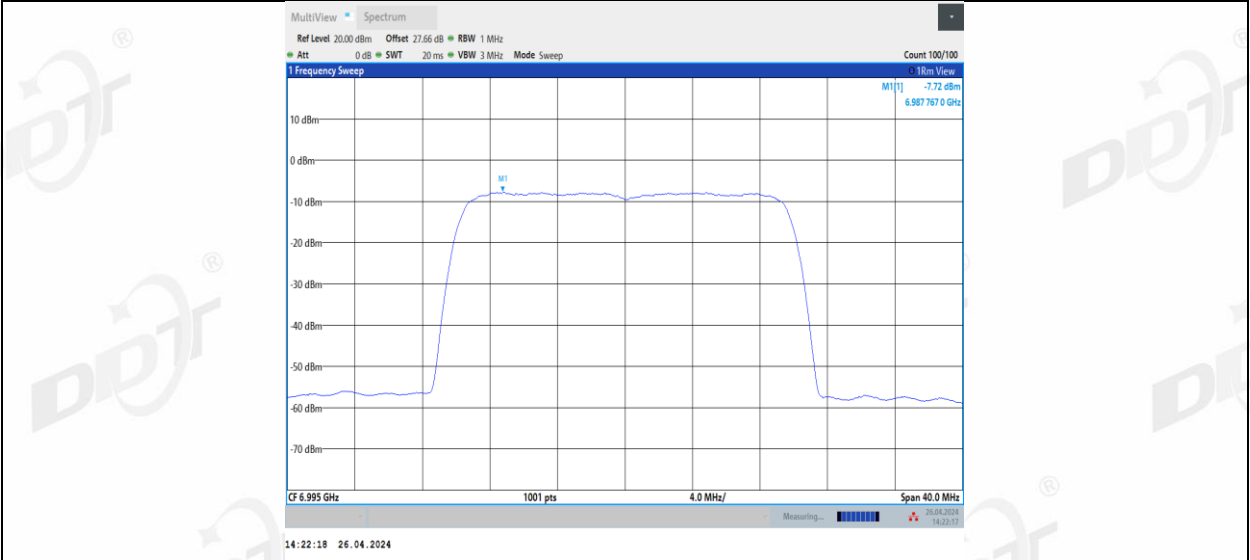
11BE20MIMO_Ant3_6995
