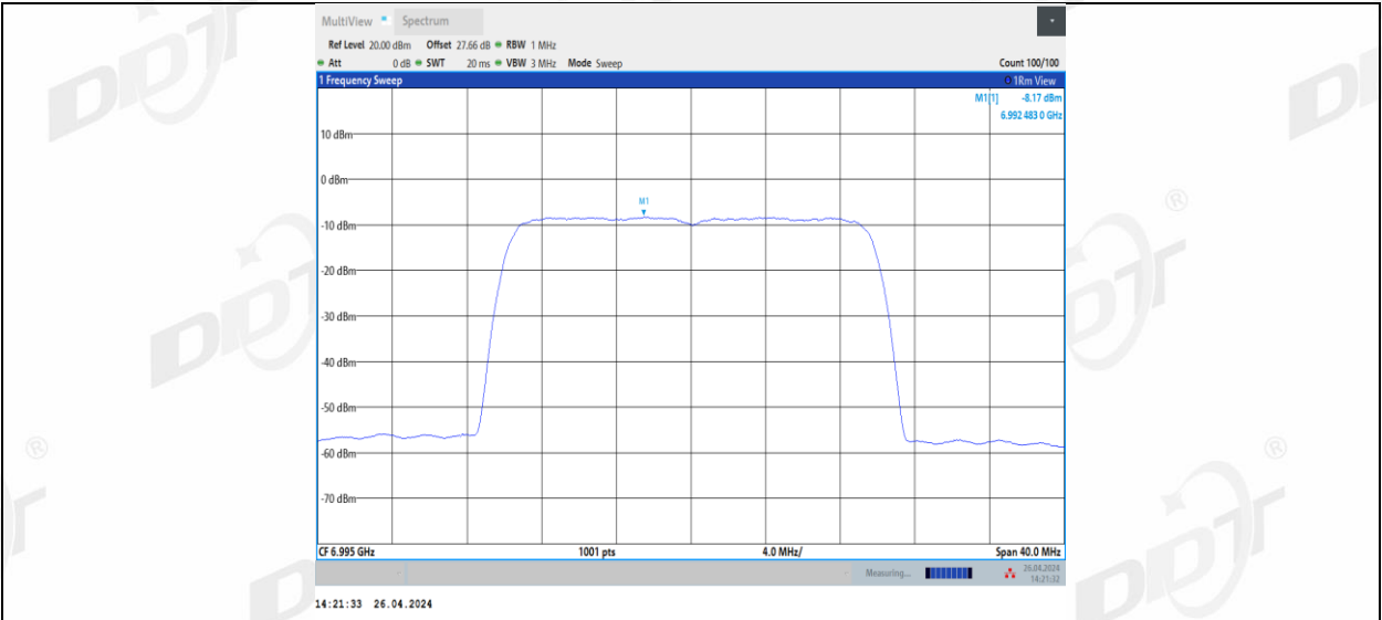
11BE20MIMO_Ant2_6995
