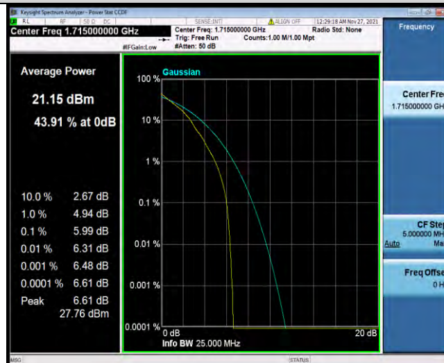
Band4-10MHz-QPSK-20000-50RB#0
