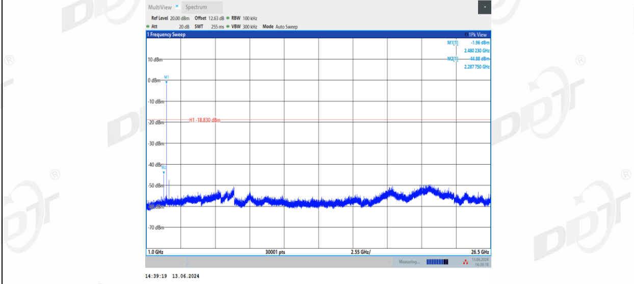
3DH5_Right side_2480_1000~26500
