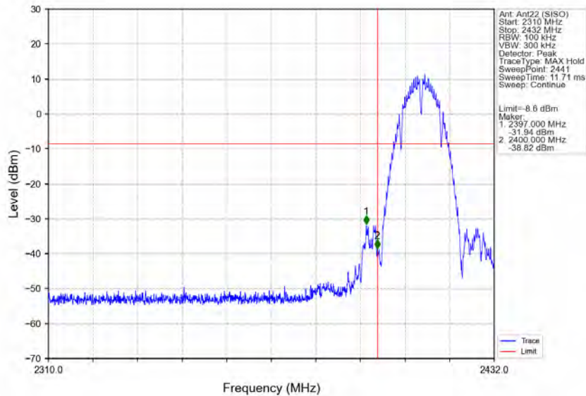
802.11b_LCH_2412MHz_Ant22 (SISO)_NTNV
