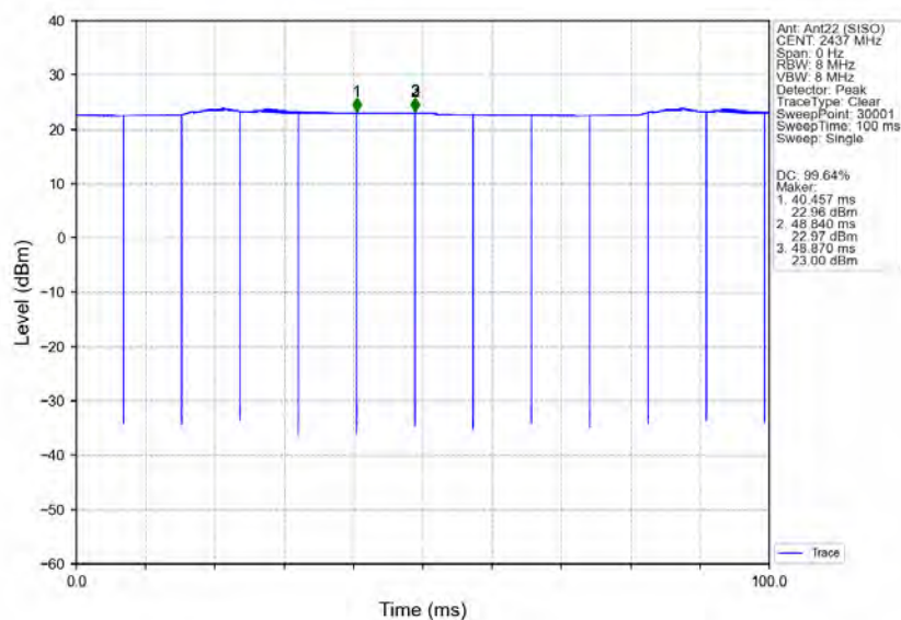
802.11b_MCH_2437MHz_Ant22 (SISO)_NTNV
