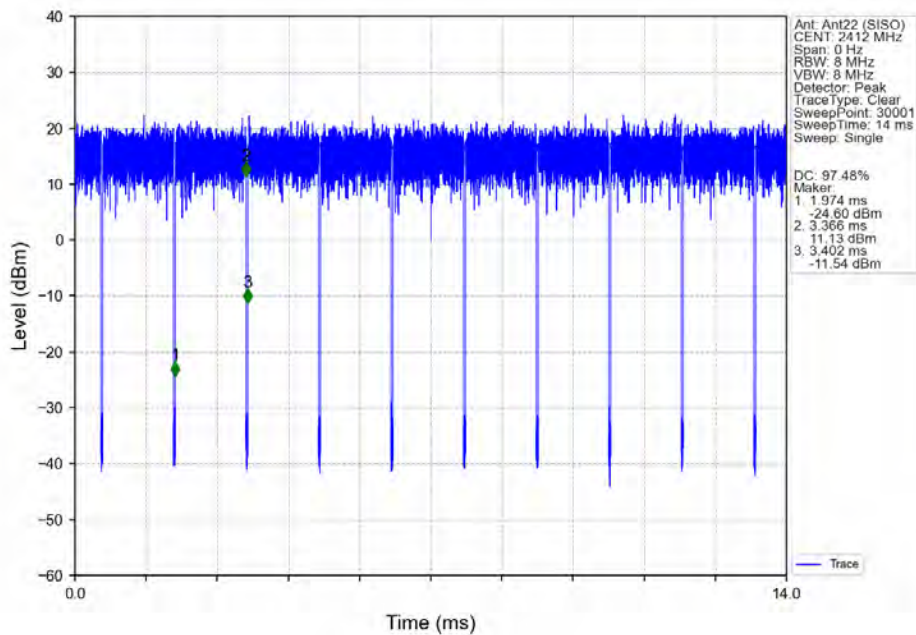
802.11g_LCH_2412MHz_Ant22 (SISO)_NTNV
