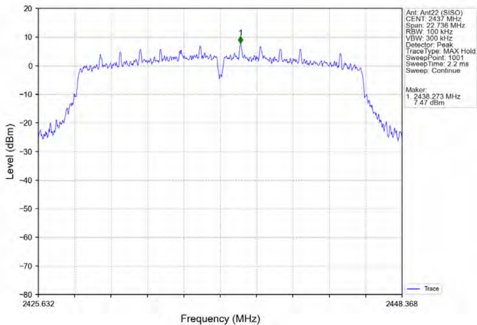
802.11ac(VHT20)_MCH_2437MHz_Ant22 (SISO)_NTNV
