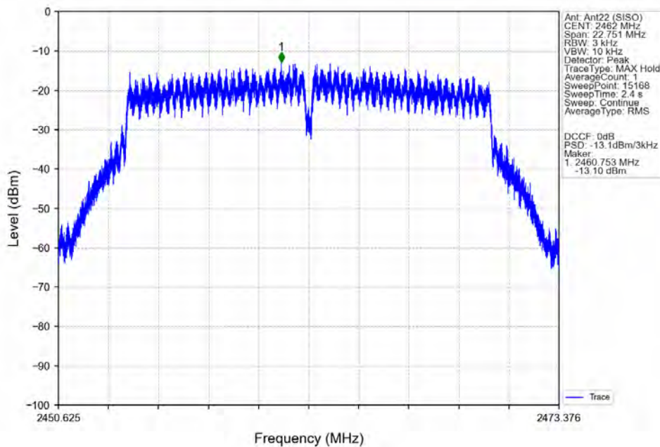
802.11g_HCH_2462MHz_Ant22 (SISO)_NTNV
