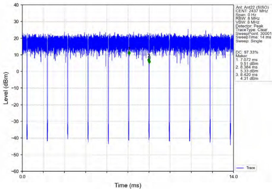
802.11ac(VHT20)_MCH_2437MHz_Ant22 (SISO)_NTNV
