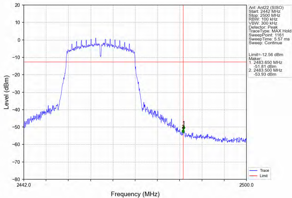
802.11n(HT20)_HCH_2462MHz_Ant22 (SISO)_NTNV
