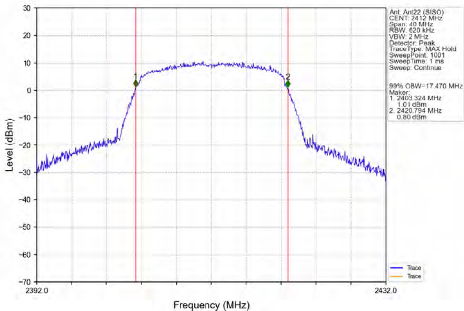
802.11g_LCH_2412MHz_Ant22 (SISO)_NTNV
