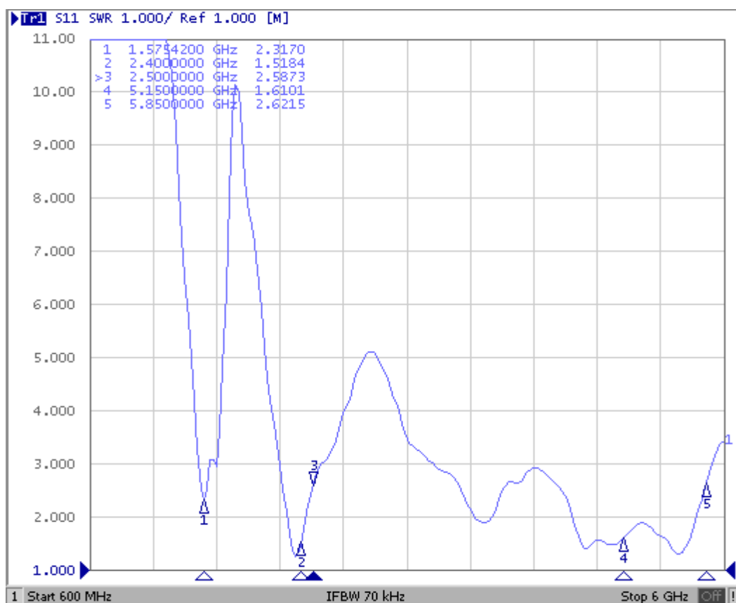
VSWR
