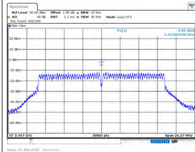
802.11n (20 MHz) / 2437 MHz
