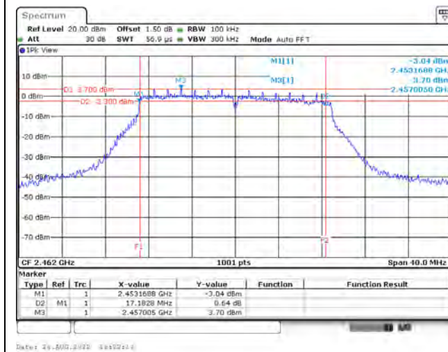
802.11n (20 MHz) / 2462 MHz
