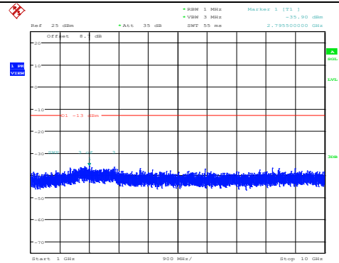
Band5-10MHz-QPSK-20525-1RB#0- Range2:1000~10000MHz
