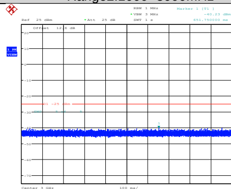
Band7-20MHz-QPSK-20850-1RB#0- Range2:1000~3000MHz
