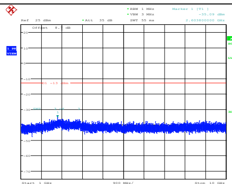
Band5-5MHz-QPSK-20525-1RB#0- Range2:1000~10000MHz
