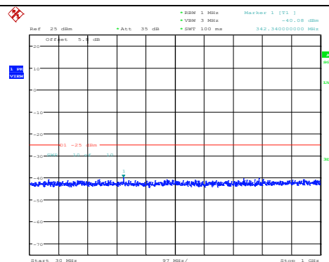
Band7-20MHz-QPSK-21350-1RB#0- Range1:30~1000MHz
