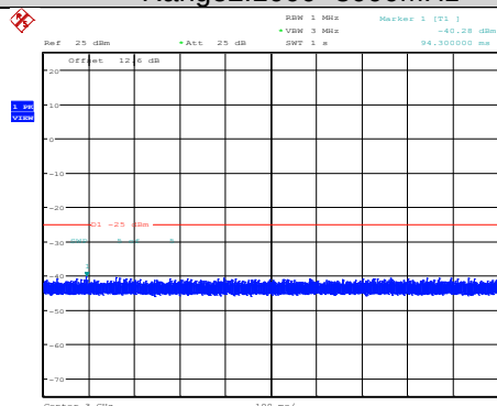
Band7-20MHz-QPSK-21100-1RB#0- Range2:1000~3000MHz
