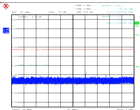
EGPRS850-128-8-30~1000MHz
