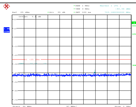
Band7-20MHz-QPSK-20850-1RB#0- Range1:30~1000MHz
