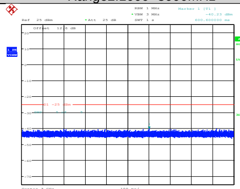
Band7-20MHz-QPSK-21350-1RB#0- Range2:1000~3000MHz
