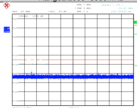
Band7-10MHz-QPSK-20800-1RB#0- Range2:1000~3000MHz
