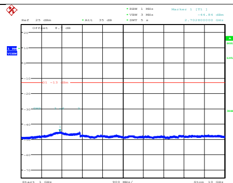
EGPRS850-190-8-1000~10000MHz
