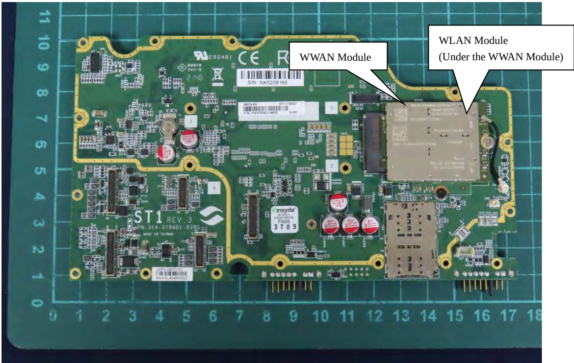
(20) EUT Photo
