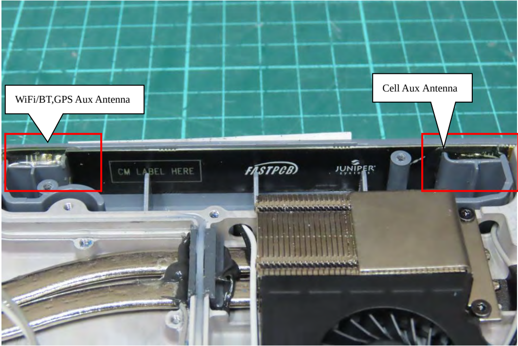
(35) EUT Photo (Aux Antenna)
