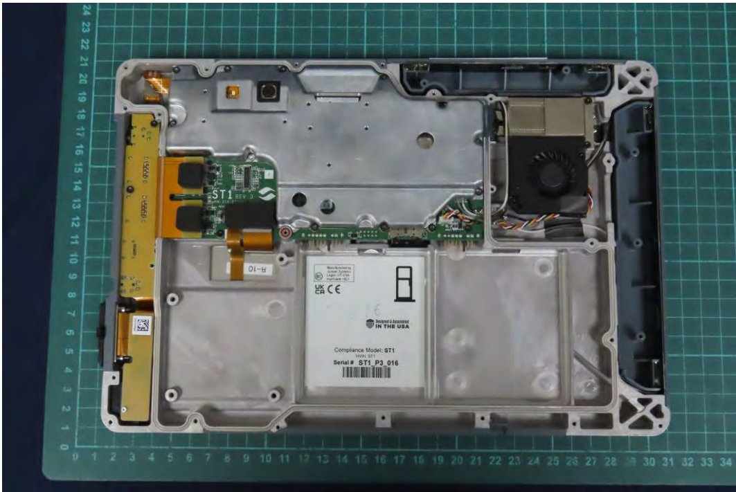
(8) EUT Photo
