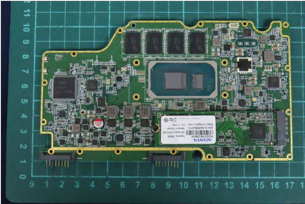
(31) EUT Photo
