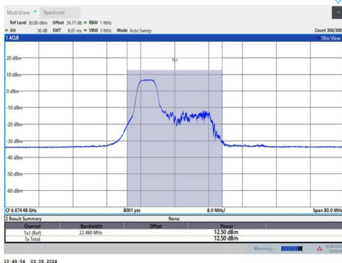
11AX40MIMO_Ant2_6685_106Tone_RU53
