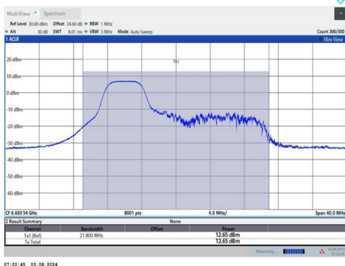
11AX20MIMO_Ant1_6695_106Tone_RU53
