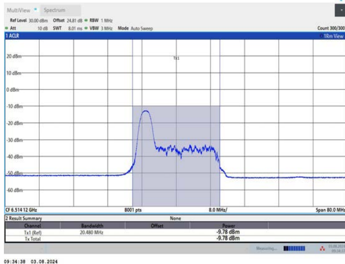
11AX40MIMO_Ant1_6525_52Tone_RU37
