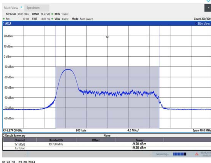
11AX20MIMO_Ant2_6875_52Tone_RU37
