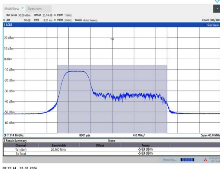
11AX20MIMO_Ant1_7115_106Tone_RU53
