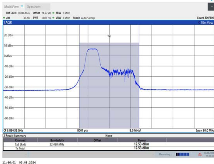
11AX40MIMO_Ant1_6845_106Tone_RU53
