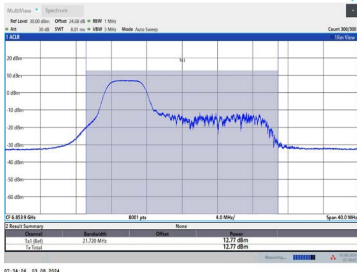
11AX20MIMO_Ant2_6855_106Tone_RU53
