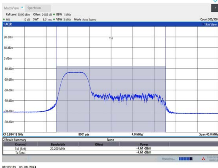
11AX20MIMO_Ant1_6995_106Tone_RU53
