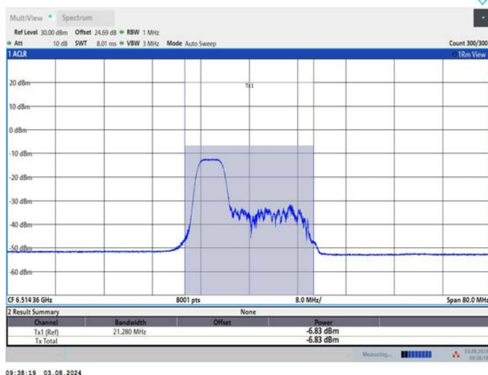
11AX40MIMO_Ant1_6525_106Tone_RU53
