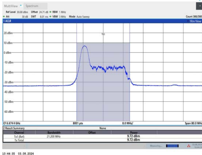
11AX40MIMO_Ant1_6685_52Tone_RU37
