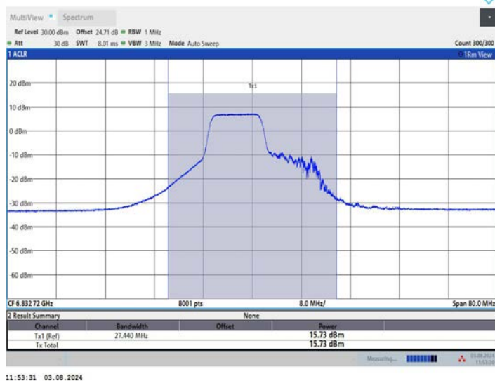
11AX40MIMO_Ant2_6845_242Tone_RU61
