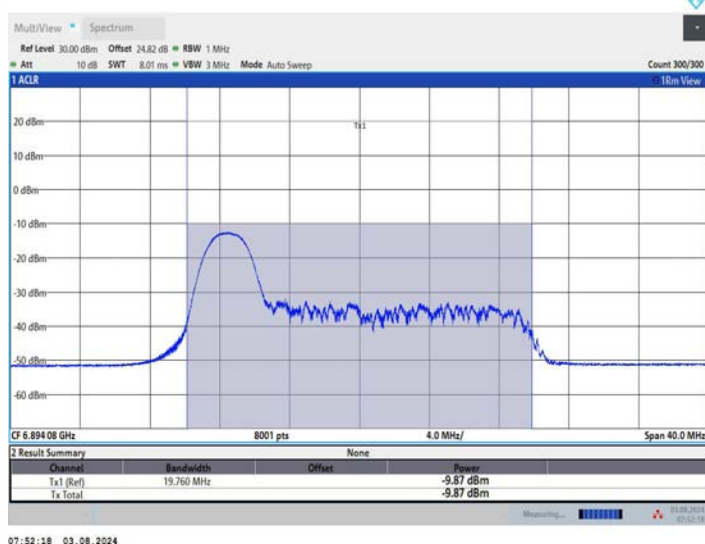
11AX20MIMO_Ant2_6895_52Tone_RU37
