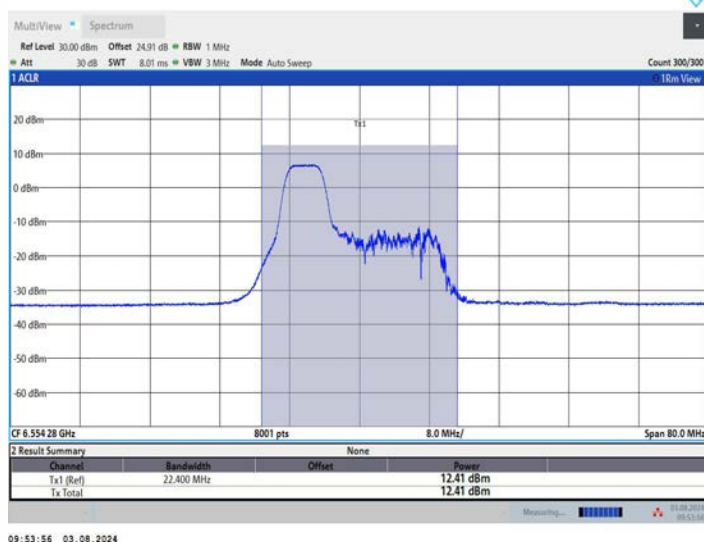
11AX40MIMO_Ant2_6565_106Tone_RU53
