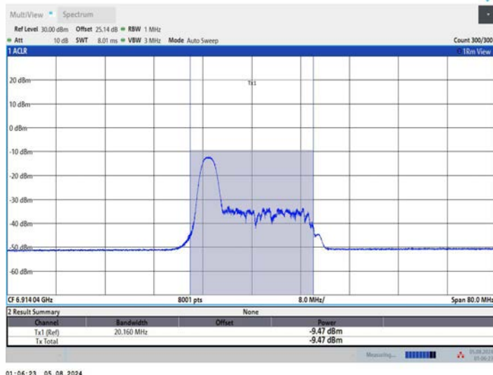
11AX40MIMO_Ant2_6925_52Tone_RU37
