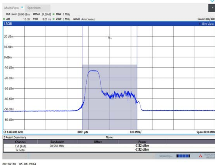
11AX40MIMO_Ant2_6885_106Tone_RU53
