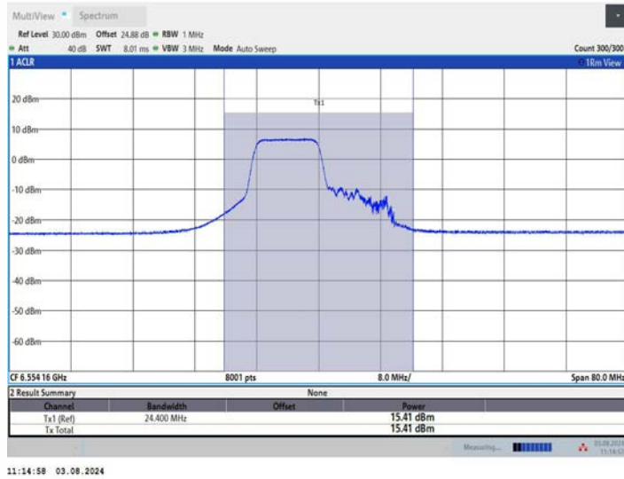
11AX40MIMO_Ant1_6565_242Tone_RU61
