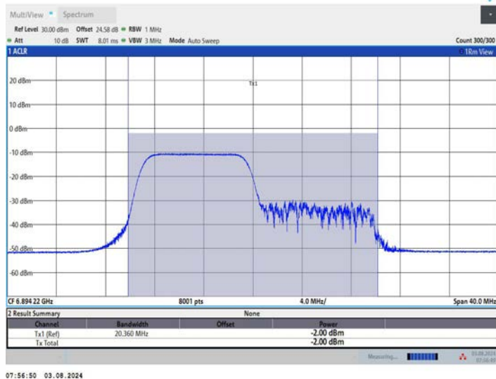
11AX20MIMO_Ant2_6895_26Tone_RU0
