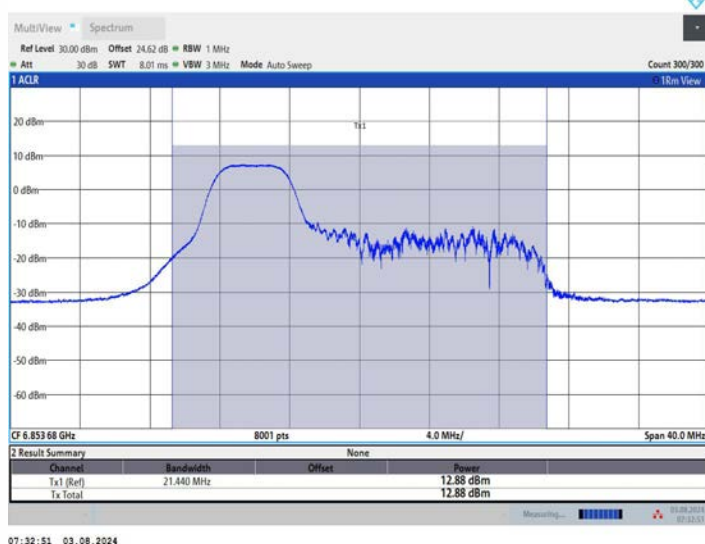
11AX20MIMO_Ant1_6855_106Tone_RU53
