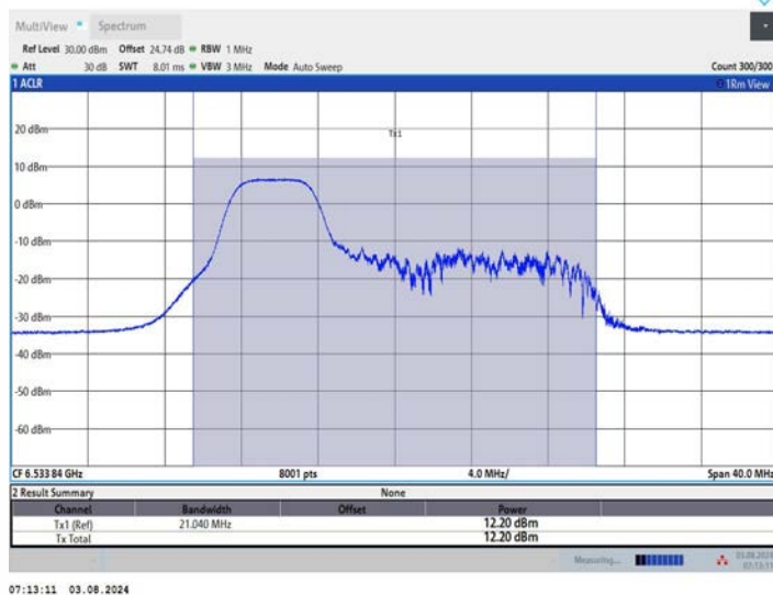
11AX20MIMO_Ant1_6535_106Tone_RU53
