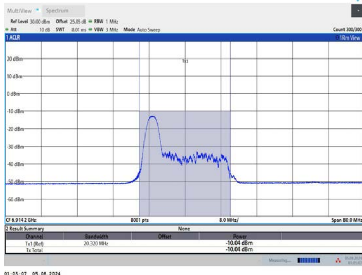
11AX40MIMO_Ant1_6925_52Tone_RU37
