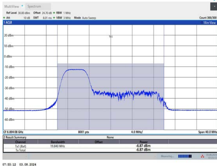
11AX20MIMO_Ant2_6895_106Tone_RU53
