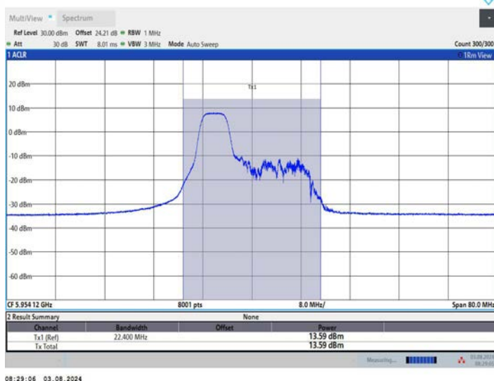
11AX40MIMO_Ant2_5965_106Tone_RU53
