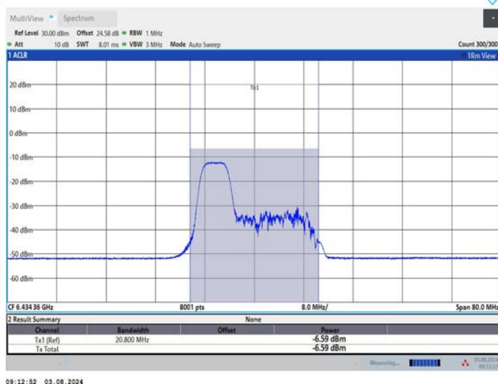
11AX40MIMO_Ant2_6445_106Tone_RU53
