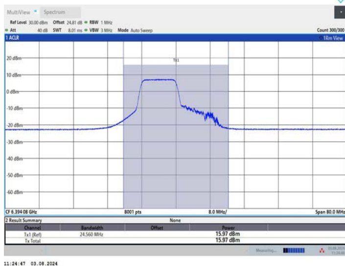
11AX40MIMO_Ant1_6405_242Tone_RU61
