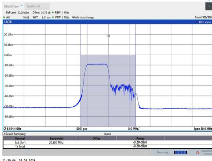
11AX40MIMO_Ant2_6525_242Tone_RU61
