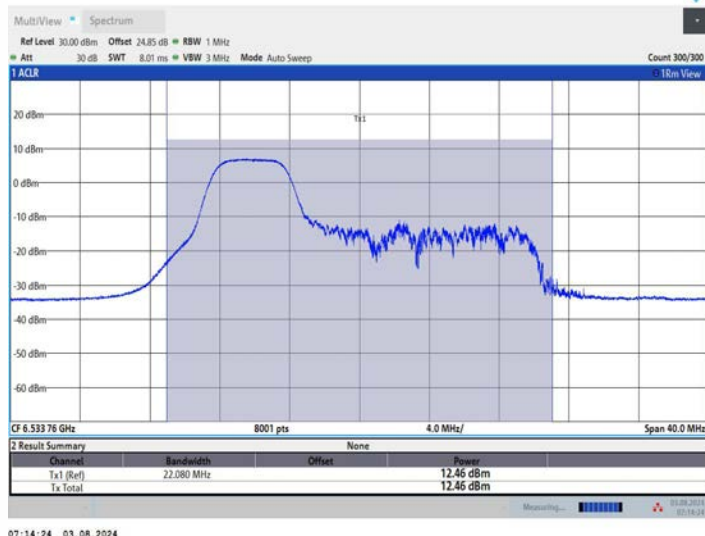
11AX20MIMO_Ant2_6535_106Tone_RU53
