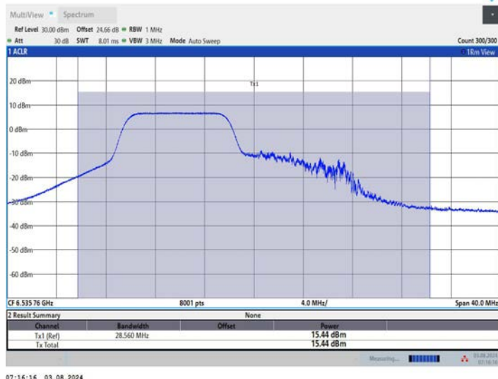
11AX20MIMO_Ant2_6535_26Tone_RU0
