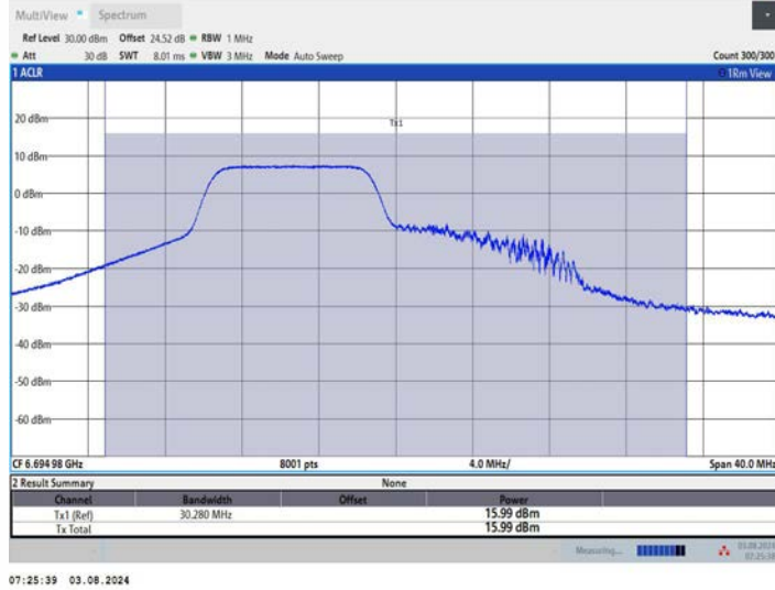
11AX20MIMO_Ant2_6695_26Tone_RU0
