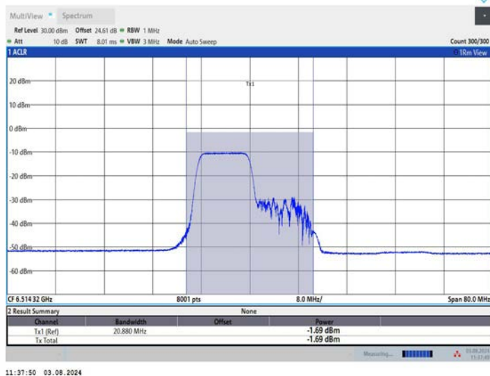
11AX40MIMO_Ant1_6525_242Tone_RU61
