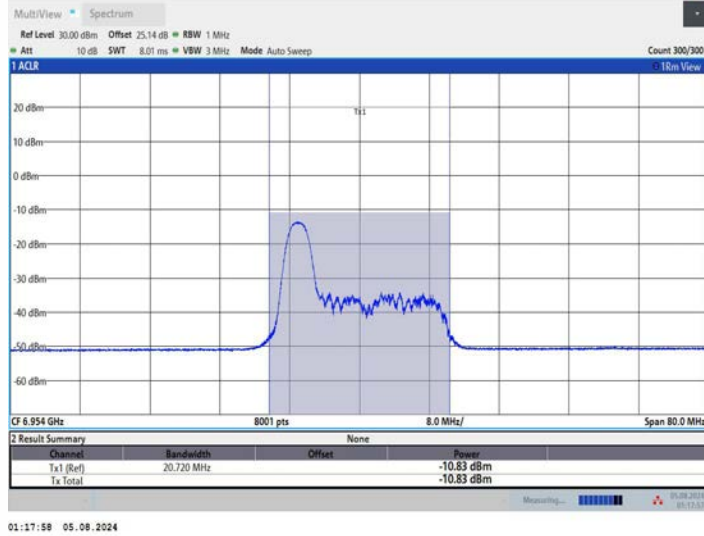
11AX40MIMO_Ant1_6965_52Tone_RU37
