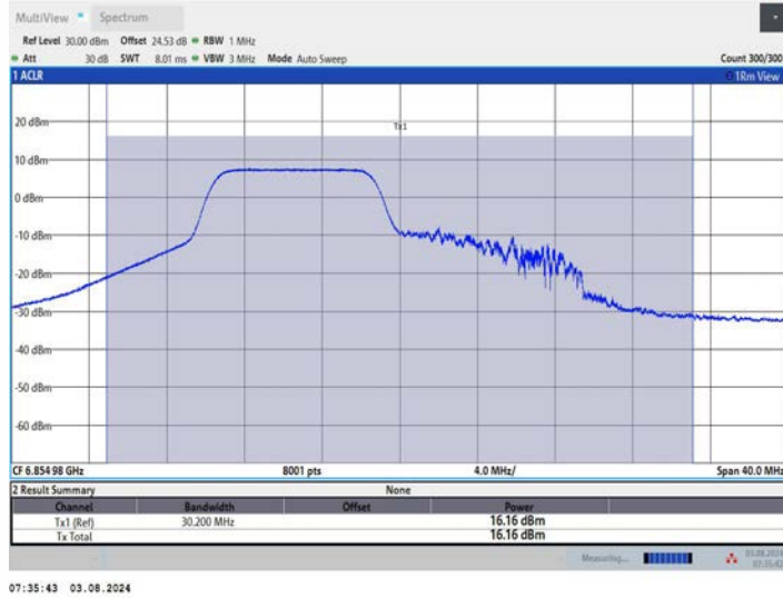
11AX20MIMO_Ant2_6855_26Tone_RU0
