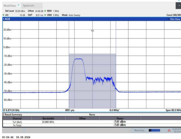
11AX40MIMO_Ant1_6885_106Tone_RU53
