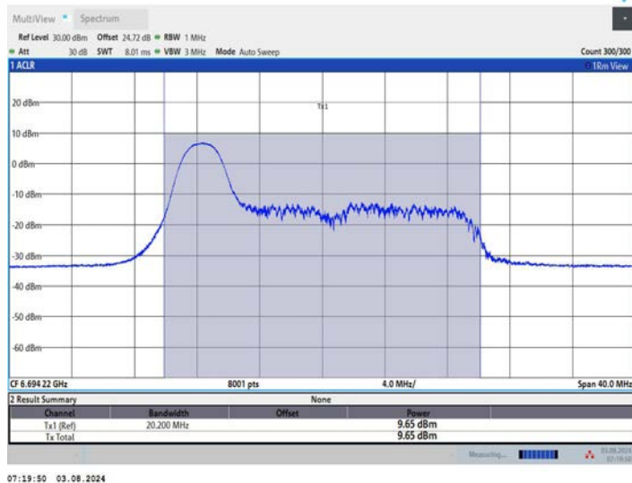
11AX20MIMO_Ant1_6695_52Tone_RU37
