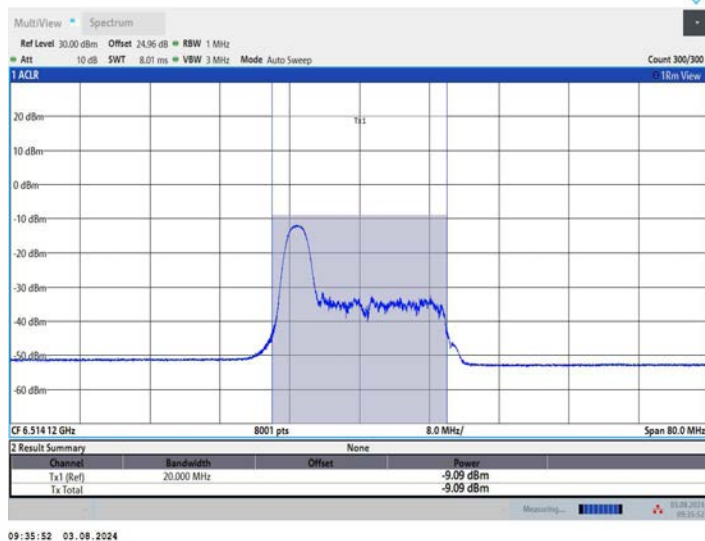
11AX40MIMO_Ant2_6525_52Tone_RU37
