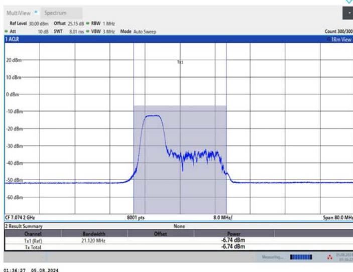
11AX40MIMO_Ant1_7085_106Tone_RU53
