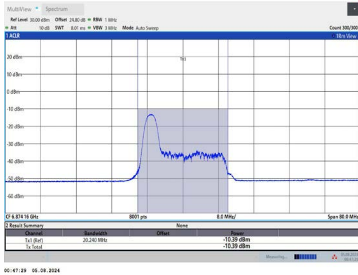
11AX40MIMO_Ant1_6885_52Tone_RU37
