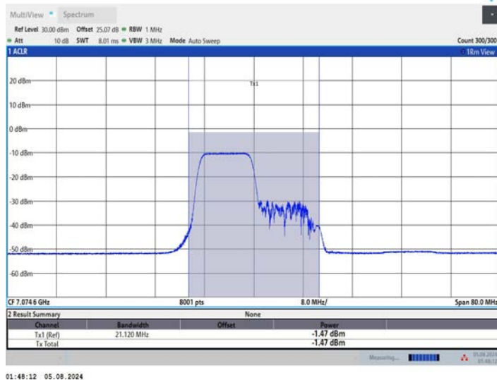
11AX40MIMO_Ant1_7085_242Tone_RU61
