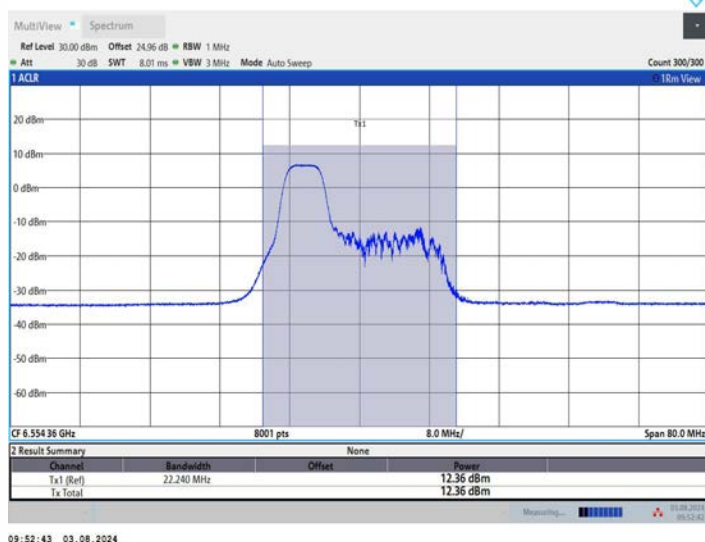
11AX40MIMO_Ant1_6565_106Tone_RU53
