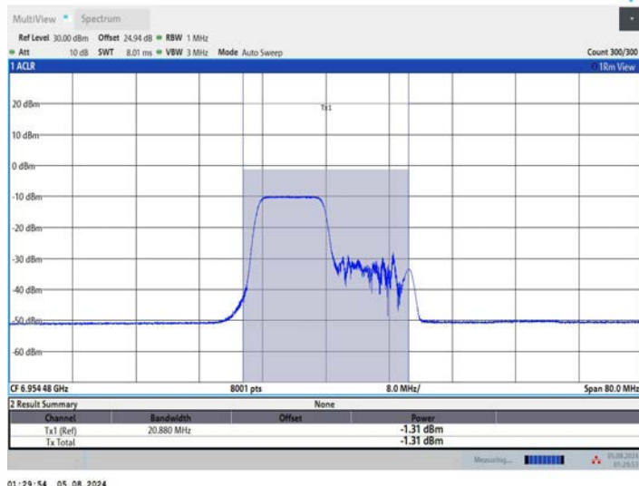
11AX40MIMO_Ant2_6965_242Tone_RU61
