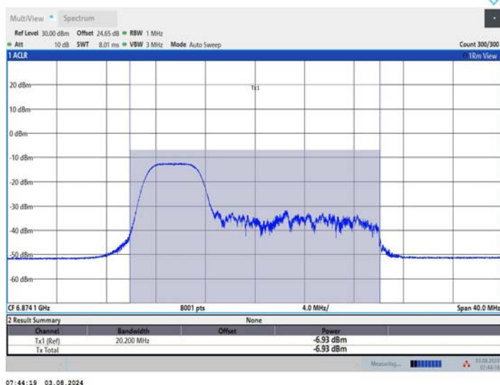
11AX20MIMO_Ant1_6875_106Tone_RU53
