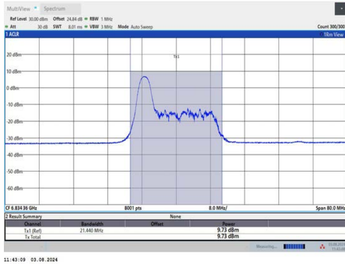
11AX40MIMO_Ant1_6845_52Tone_RU37
