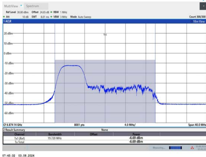
11AX20MIMO_Ant2_6875_106Tone_RU53
