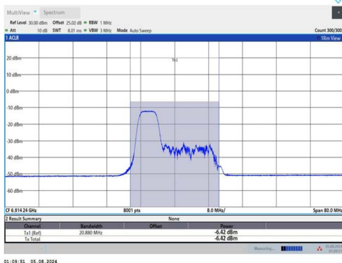
11AX40MIMO_Ant2_6925_106Tone_RU53
