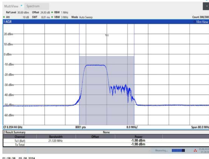
11AX40MIMO_Ant1_6965_242Tone_RU61
