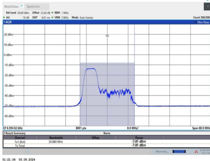
11AX40MIMO_Ant1_6965_106Tone_RU53
