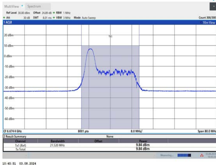
11AX40MIMO_Ant2_6685_52Tone_RU37
