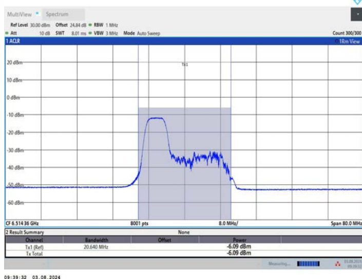
11AX40MIMO_Ant2_6525_106Tone_RU53
