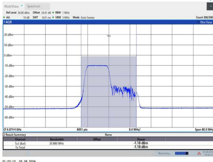
11AX40MIMO_Ant2_6885_242Tone_RU61
