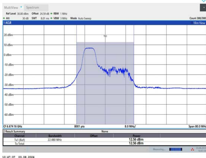
11AX40MIMO_Ant1_6685_106Tone_RU53
