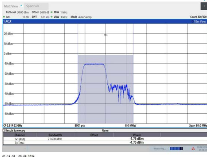
11AX40MIMO_Ant1_6925_242Tone_RU61
