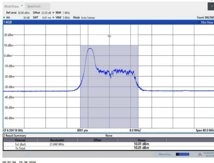
11AX40MIMO_Ant2_6565_52Tone_RU37
