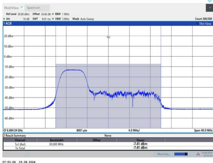
11AX20MIMO_Ant1_6895_106Tone_RU53
