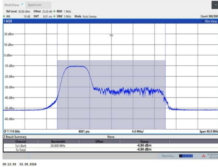
11AX20MIMO_Ant2_7115_106Tone_RU53
