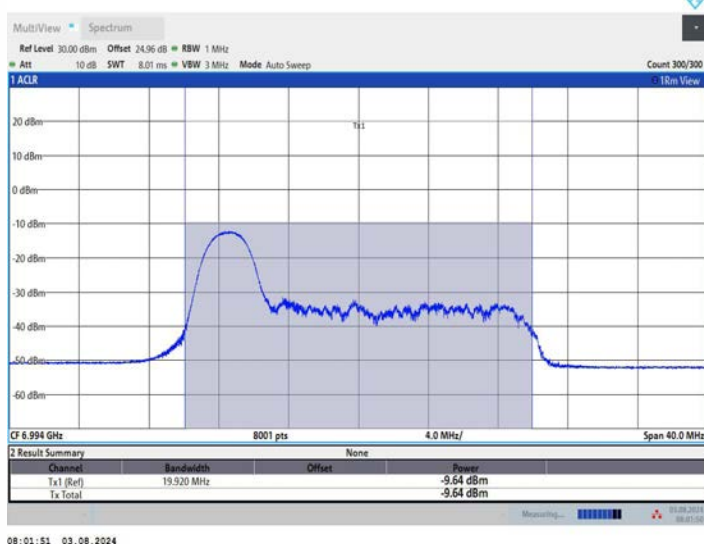
11AX20MIMO_Ant2_6995_52Tone_RU37
