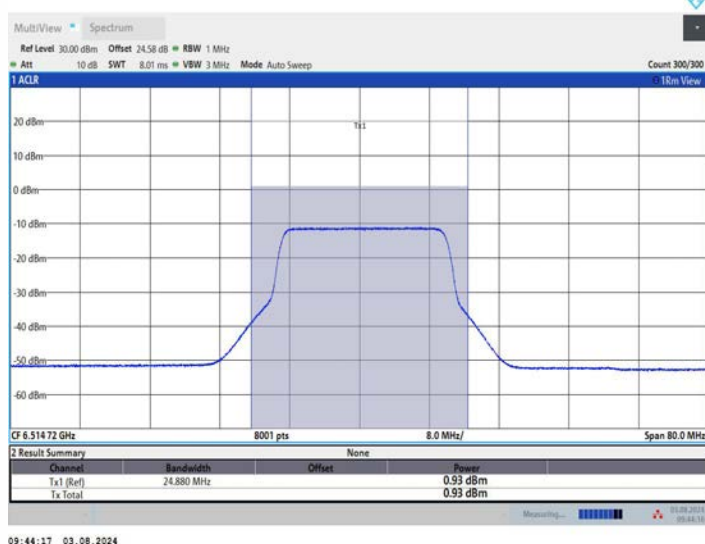
11AX40MIMO_Ant2_6525_26Tone_RU0
