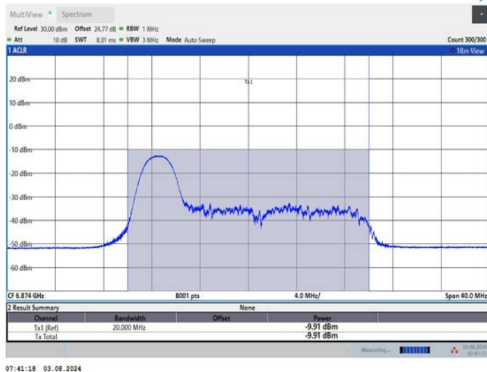
11AX20MIMO_Ant1_6875_52Tone_RU37
