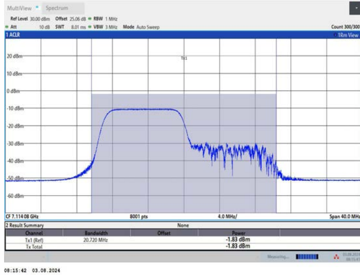
11AX20MIMO_Ant2_7115_26Tone_RU0
