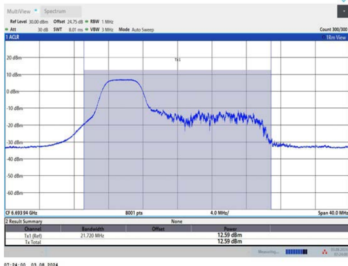
11AX20MIMO_Ant2_6695_106Tone_RU53
