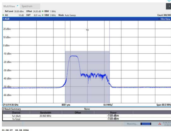
11AX40MIMO_Ant1_6925_106Tone_RU53
