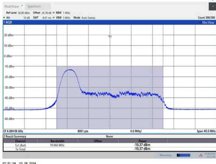
11AX20MIMO_Ant1_6895_52Tone_RU37
