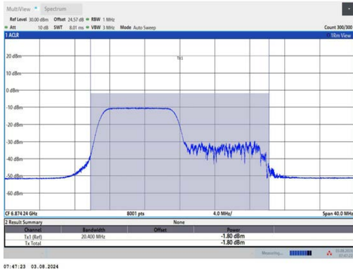
11AX20MIMO_Ant2_6875_26Tone_RU0
