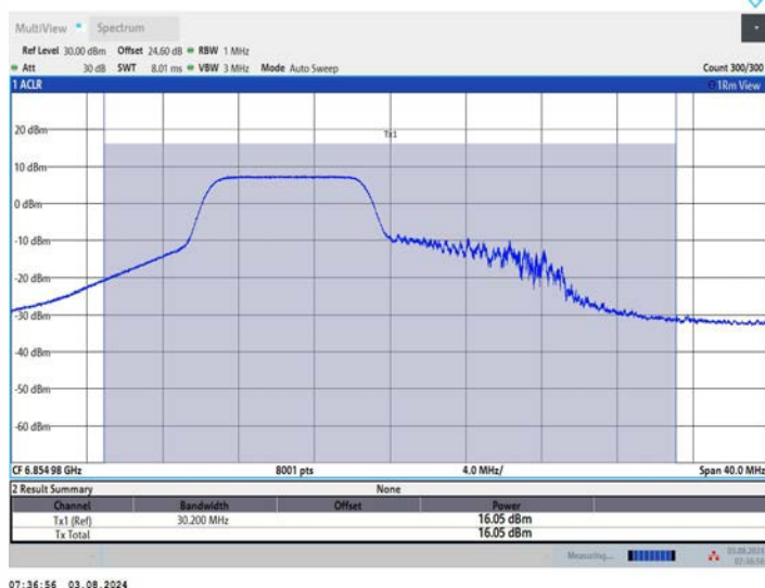
11AX20MIMO_Ant1_6875_26Tone_RU0
