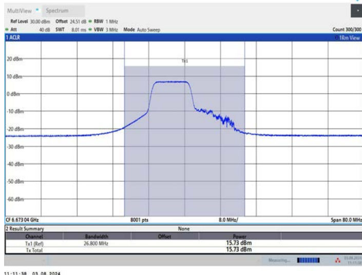
11AX40MIMO_Ant1_6685_242Tone_RU61
