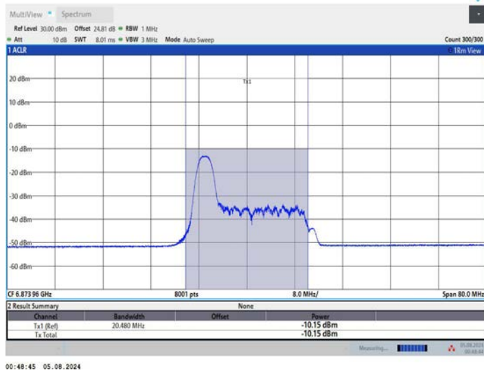
11AX40MIMO_Ant2_6885_52Tone_RU37
