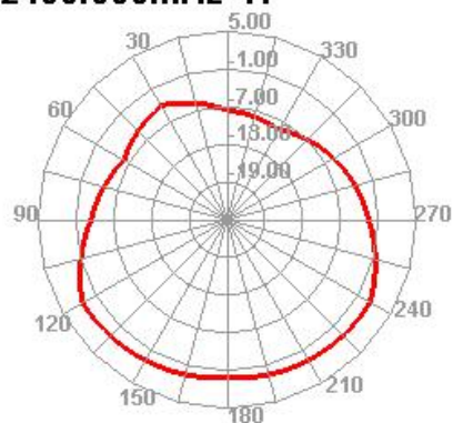
2400.000MHz H
