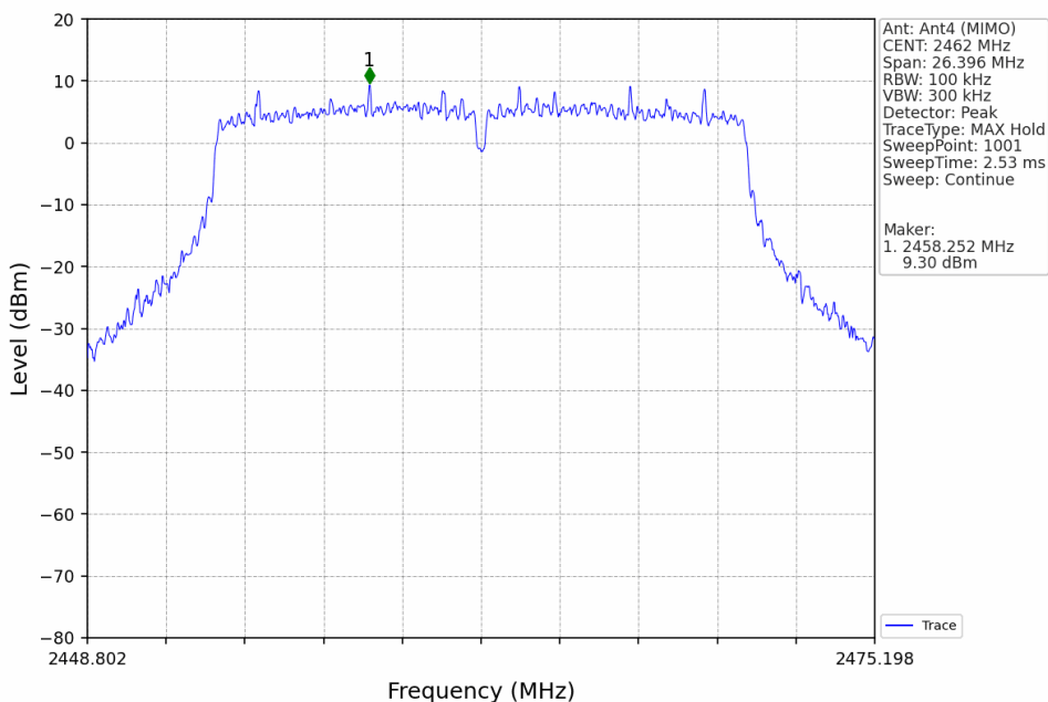
802.11n(HT20)_HCH_2462MHz_Ant4 (MIMO)_NTNV
