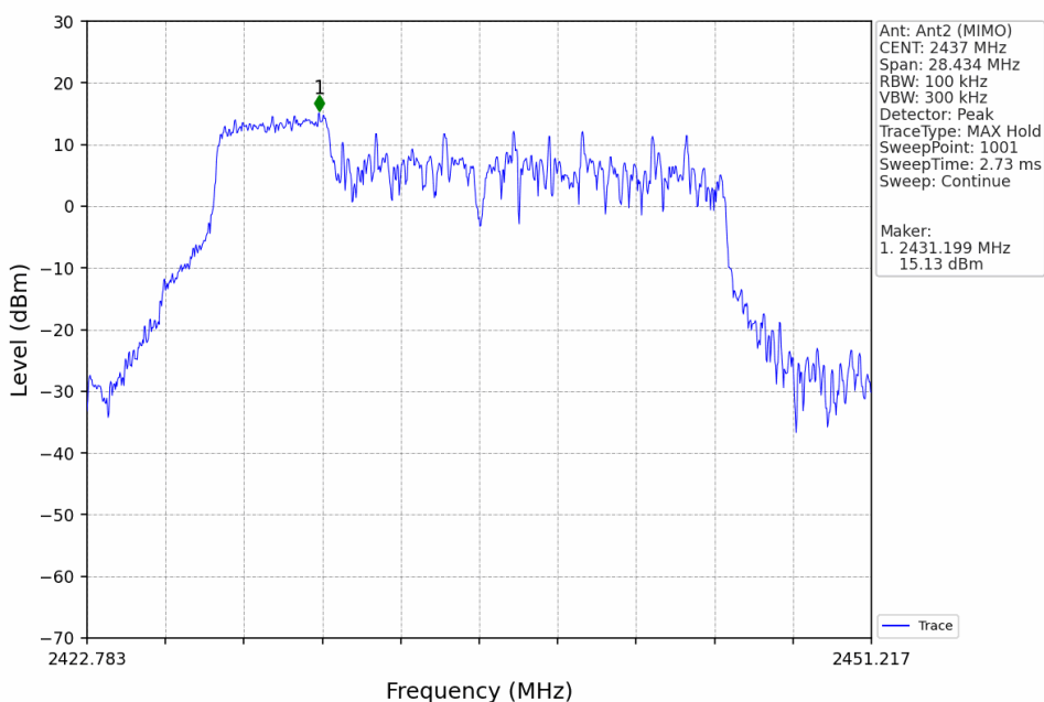
802.11ax(HEW20)_MCH_2437MHz_RU52_Left_Ant2 (MIMO)_NTNV
