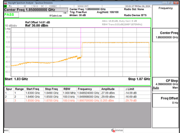
Band2 20MHz CP_OFDM_SCS15kHz QPSK RB1_0 CH372000
