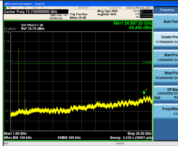
BLE 2M_2480_0~Reference
