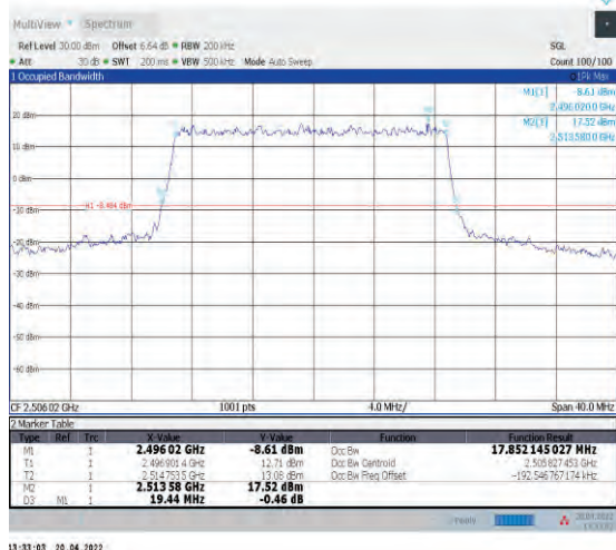
1-N41--30-20-L-1-DFT-QPSK-Outer_Full-50@0-Ant1 -17.852-19.440≤20-PASS
