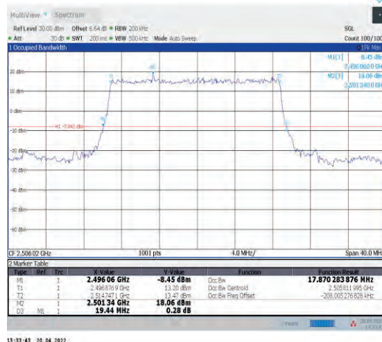
1-N41--30-20-L-2-DFT-PI2BPSK-Outer_Full-50@0-A nt1-17.87-19.440≤20-PASS
