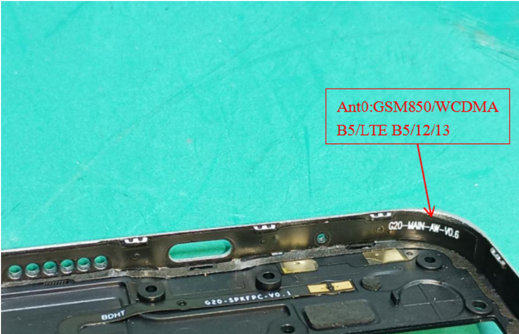
Ant0
