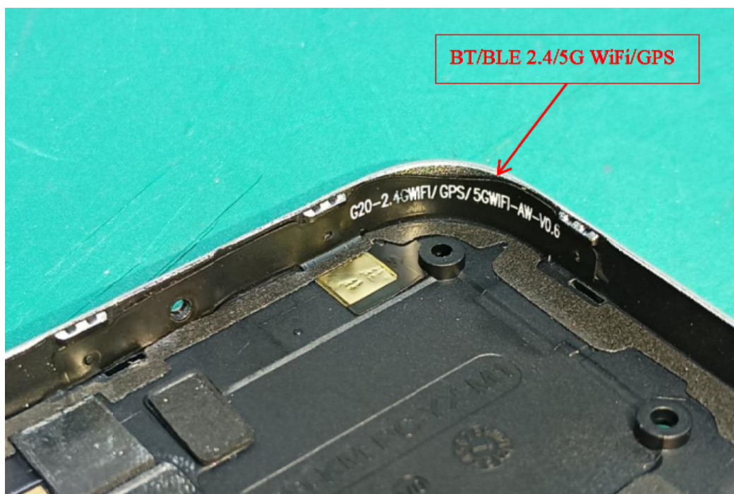
BT/Wi-Fi/GPS ANT
