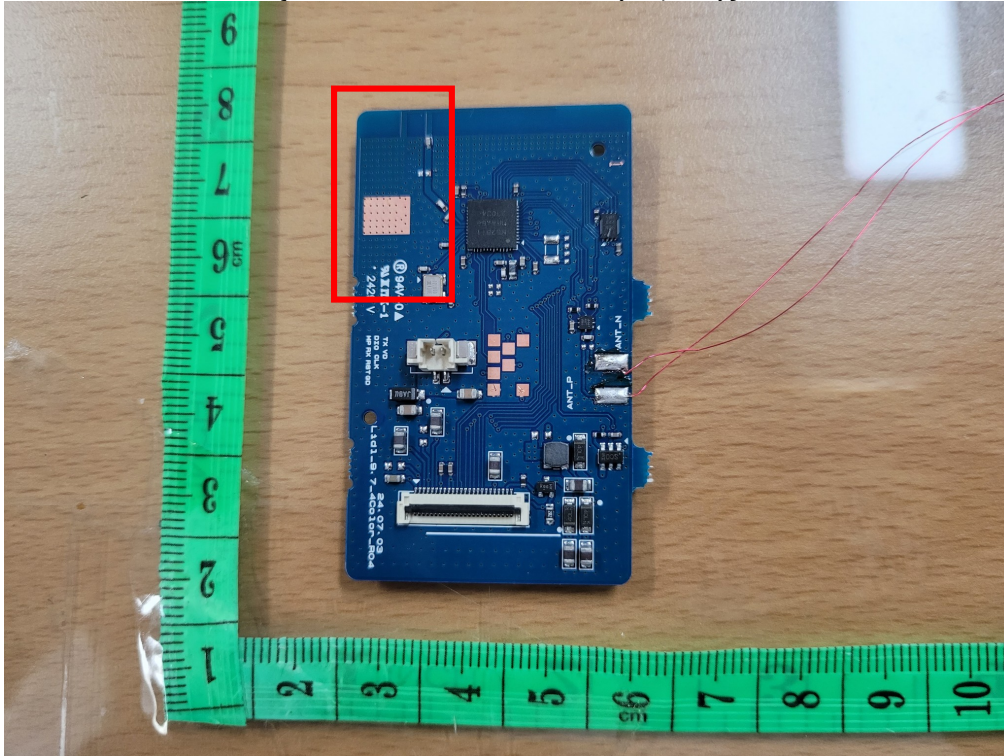
{NFC Antenna(RX)}
