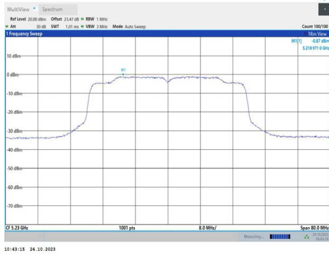
11AX40MIMO_Ant2_5230
