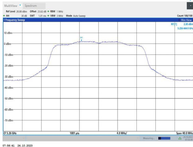
11AX20MIMO_Ant2_5260
