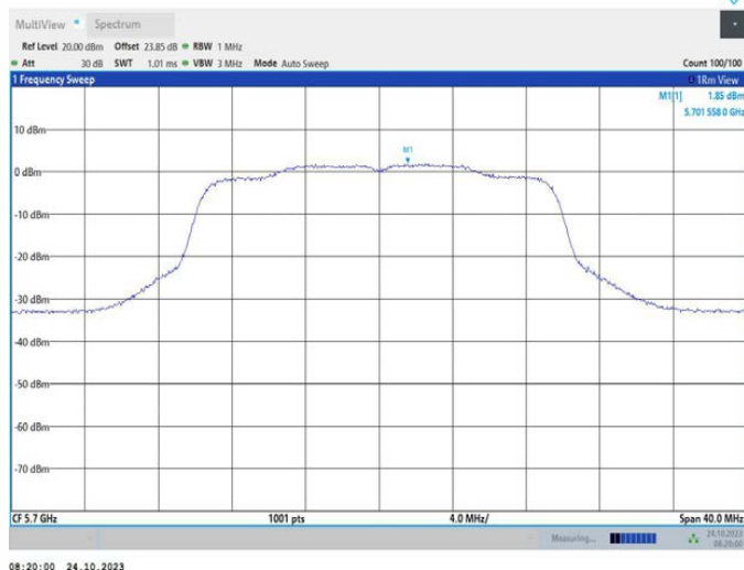
11AX20MIMO_Ant1_5700
