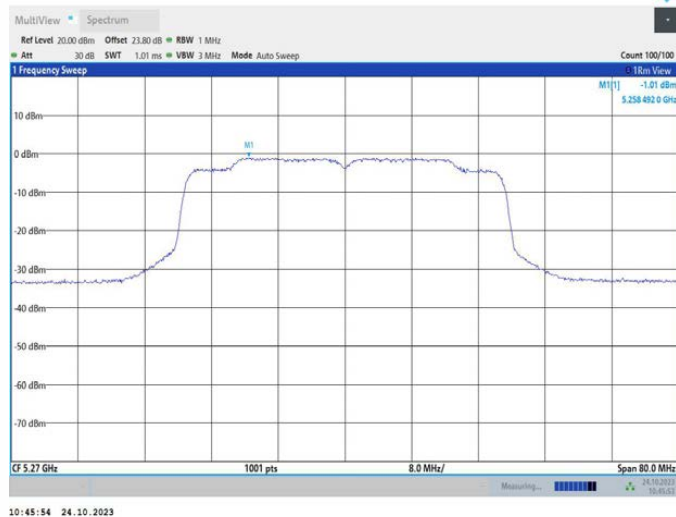
11AX40MIMO_Ant1_5270
