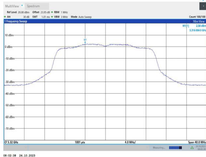
11AX20MIMO_Ant1_5320
