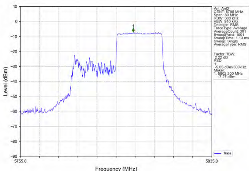
802.11ax(HE40) HCH 5795MHz RU242 Right MIMO NTN
