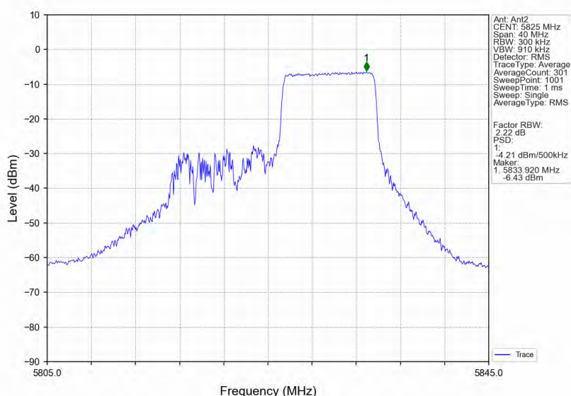
802.11ax(HE20) HCH 5825MHz RU106 Right MIMO NTN
