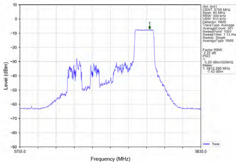
802.11ax(HE40) HCH 5795MHz RU106 Right Ant1 NTV
