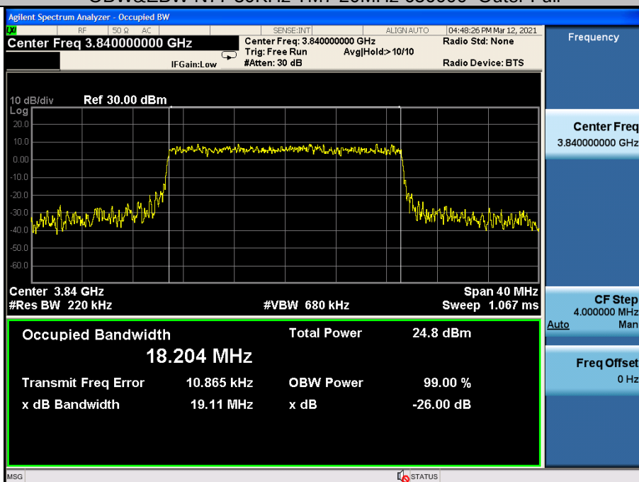
OBW&amp;EBW N77 30KHz TM8 20MHz 656000 Outer Full
