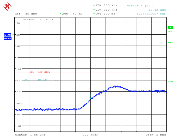
Band2-5MHz-QPSK-18625-1RB#24
