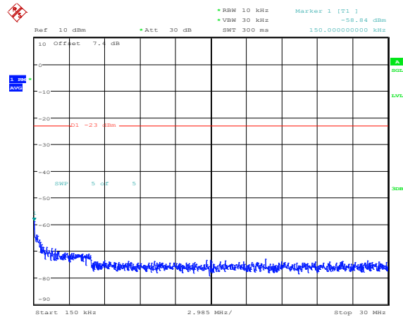
Band2-1.4MHz-QPSK-18900-1RB#0-Range2:0.15~30MHz
