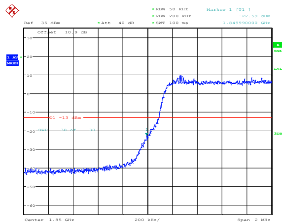
Band2-3MHz-QPSK-18615-15RB#0
