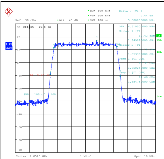
Band2-5MHz-QPSK-18625-25RB#0-PASS
