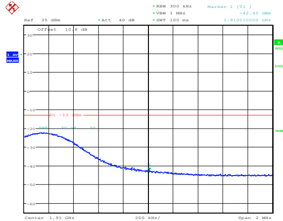
Band2-15MHz-16QAM-19125-1RB#74
