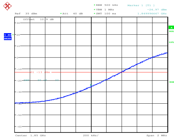
Band2-20MHz-QPSK-18700-100RB#0
