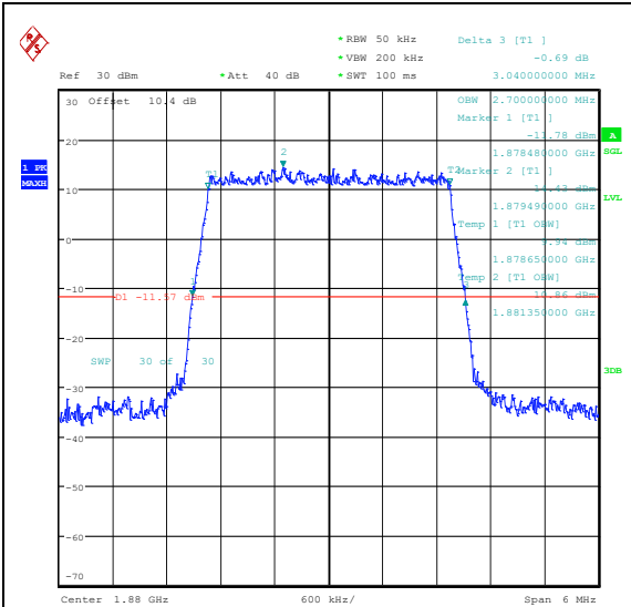
Band2-3MHz-QPSK-18900-15RB#0-PASS
