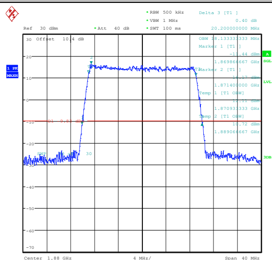
Band2-20MHz-16QAM-18700-100RB#0-PASS
