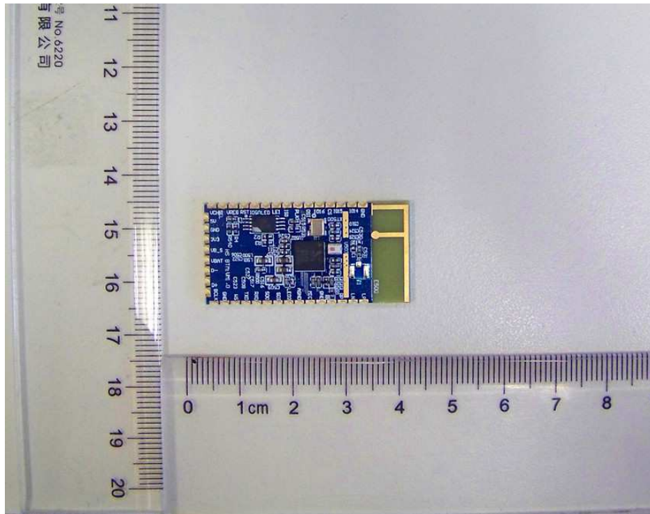
BT module
