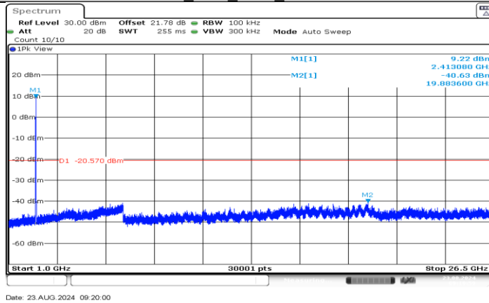
11G_Ant1_2412_1000~26500
