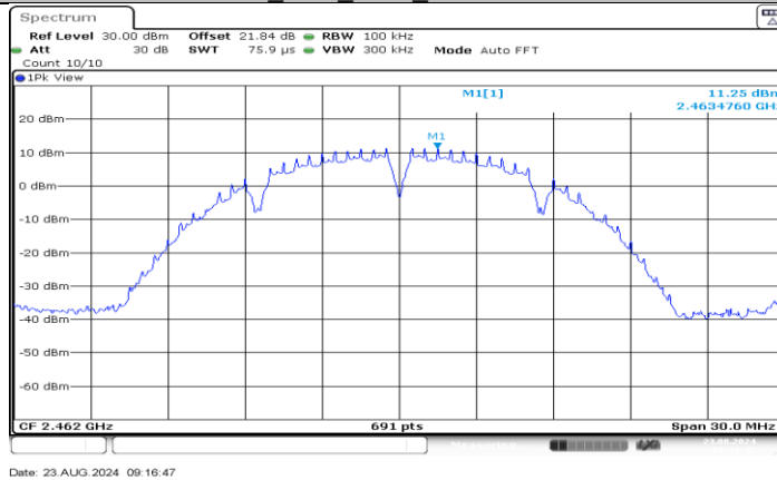
11B_Ant1_2462_0-Reference
