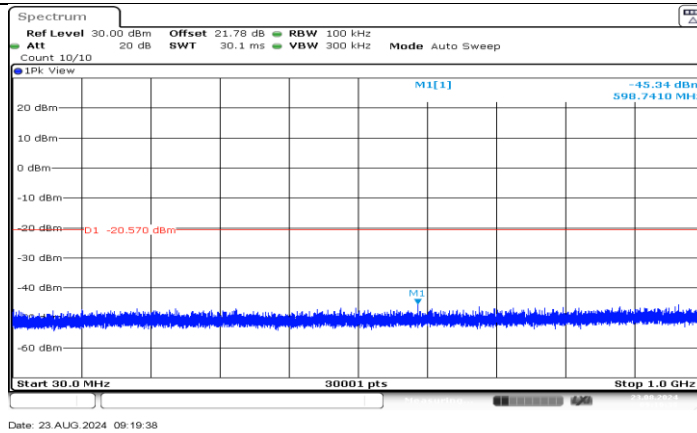
11G_Ant1_2412_30~1000
