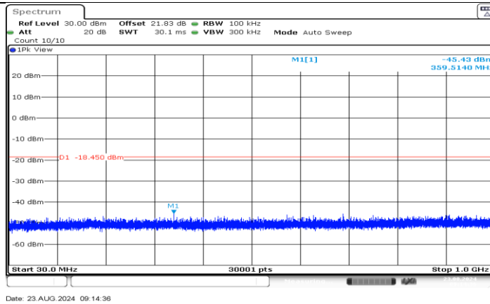
11B_Ant1_2437_30-1000
