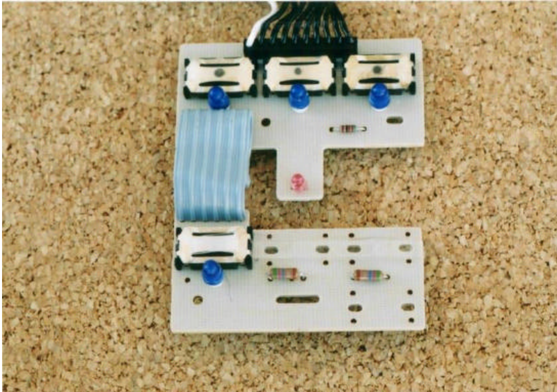
CSpSIHL3 Keypad PCB - Top
