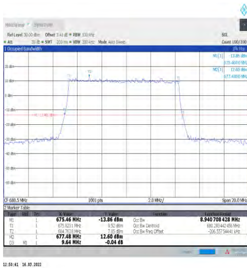
1-N71-15-10-M-3-DFT-16QAM-Outer_Full-50@0-Ant1 1-8.941-9.640≤10-PASS
