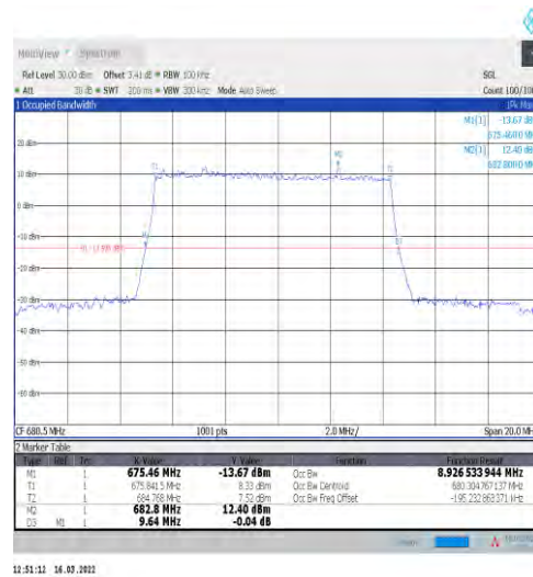
1-N71-15-10-M-4-DFT-64QAM-Outer_Full-50@0-Ant1 1-8.927-9.640≤10-PASS
