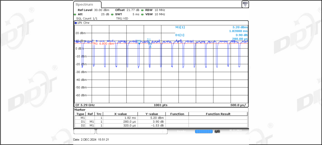
11AX80MIMO_Ant2_5290
