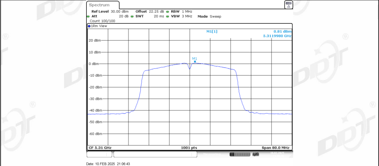
11N40MIMO_Ant2_5310
