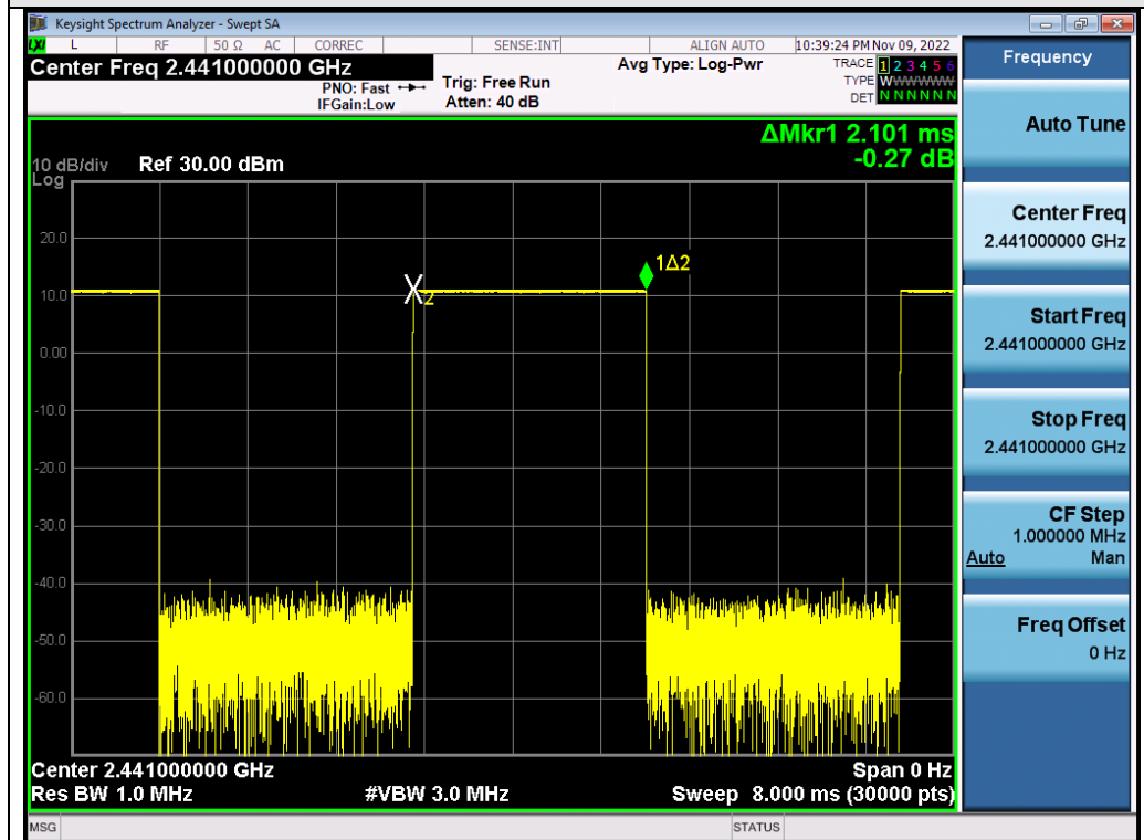
Test_Graph_2.4G_HOP_ANT2_NA_1Mbps_2441_Time per Burst
