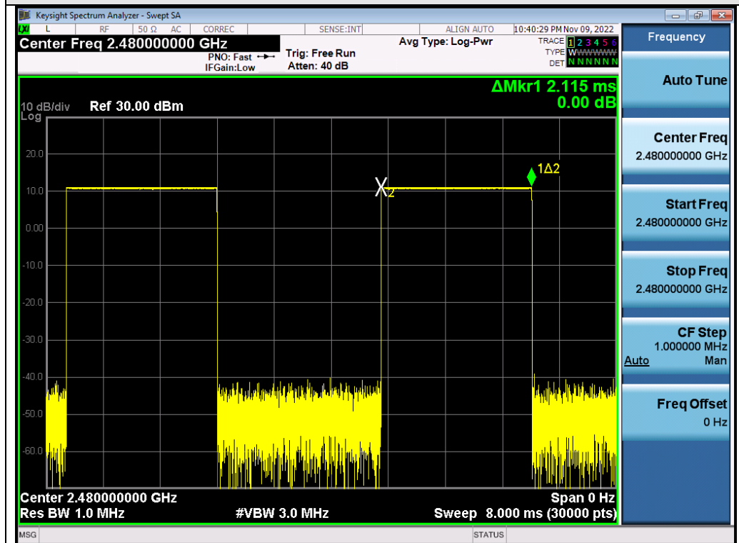
Test_Graph_2.4G_HOP_ANT2_NA_1Mbps_2480_Time per Burst
