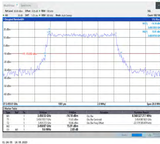
1-N78-3450-3550-PC1-30-10-L-1-DFT-QPSK-Outer_Full-24@0-Ant0-8.568-9.600-≤10-PASS
