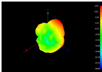
2400MHz
