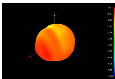
2400MHz
