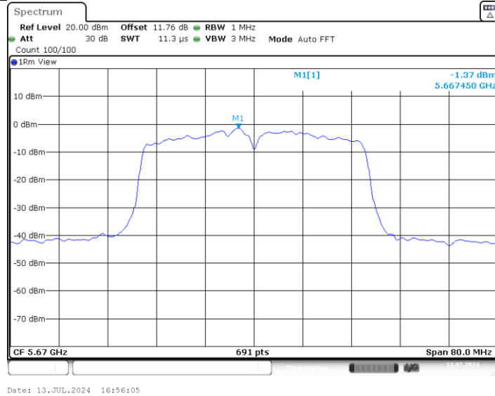
11AX40MIMO_Ant2_5670
