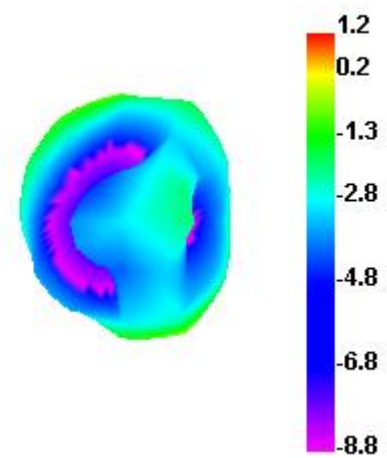
2400.000MHz
