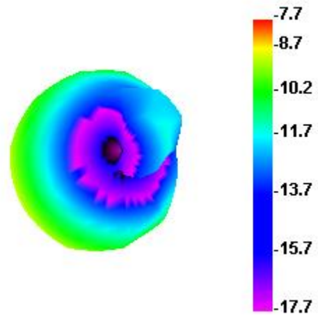
1800.000MHz
