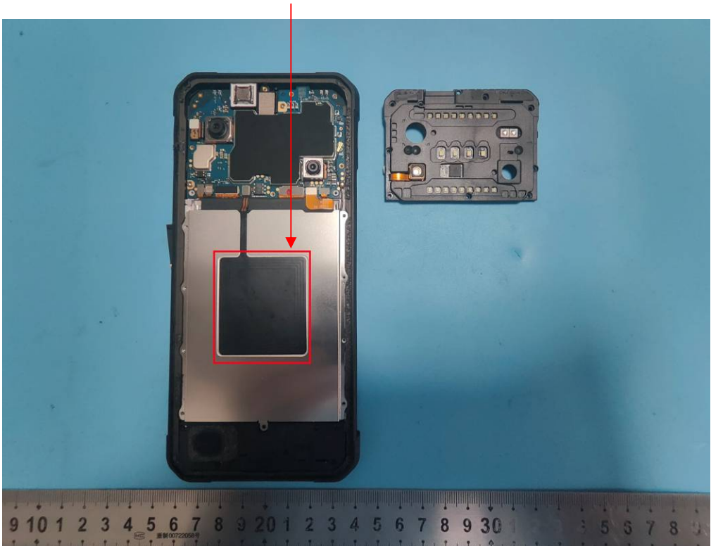
NFC Ant
