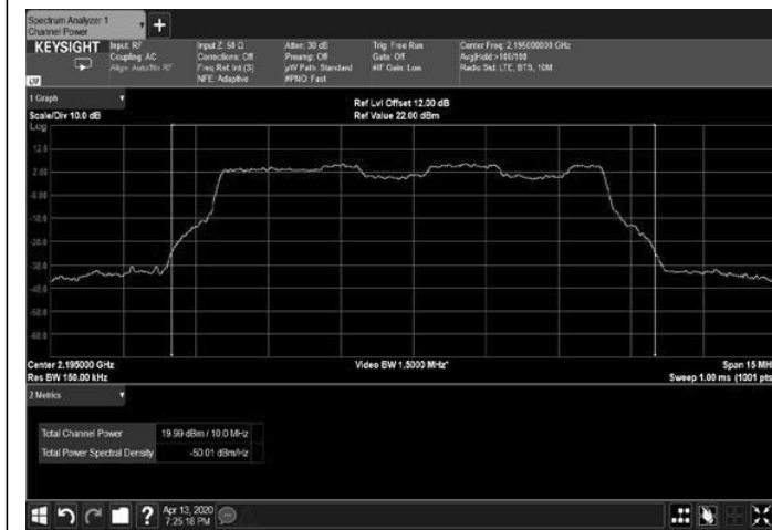
Figure 21: 16QAM 10MHz B.W.; 2195.0MHz, 60kHz
