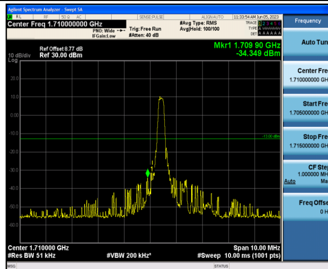
Band4-3MHz-QPSK-19965-1-0-Low--34.35-PASS
