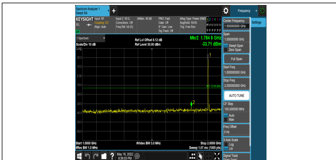
Band2-5MHz-QPSK-19175-1RB#0-Range4:1000~2000MHz
