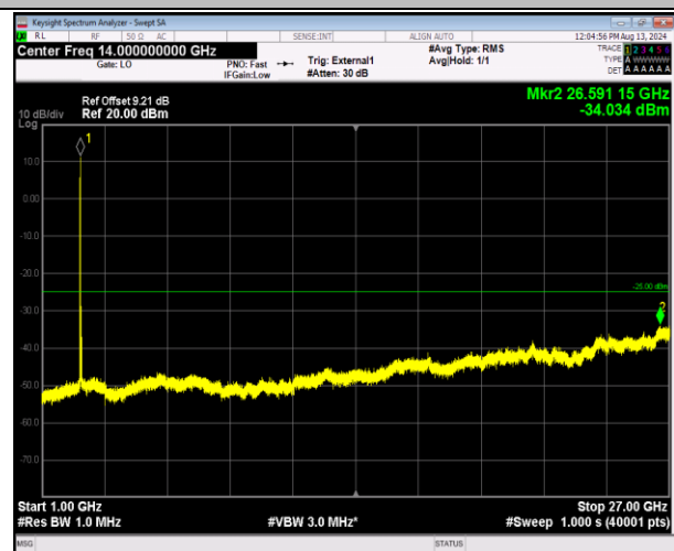
41-41-20MHz-20MHz-QPSK-QPSK-40641-40839-1RB#0- 1RB#99-1000~27000MHz-PASS
