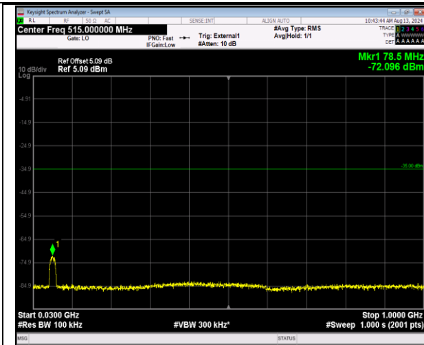
41-41-20MHz-5MHz-QPSK-QPSK-41090-41207-100RB #0-25RB#0-30~1000MHz-PASS
