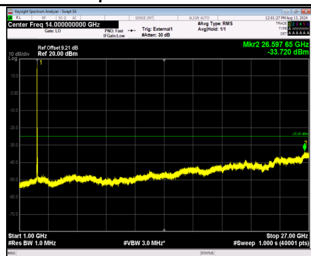
41-41-20MHz-20MHz-QPSK-QPSK-40641-40839-1RB#0- ORB#0-1000~27000MHz-PASS
