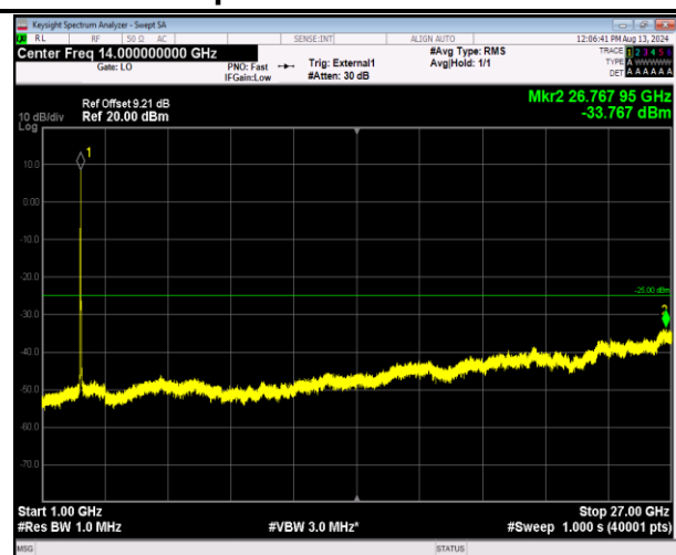
41-41-20MHz-20MHz-QPSK-QPSK-40641-40839-100RB #0-100RB#0-1000~27000MHz-PASS
