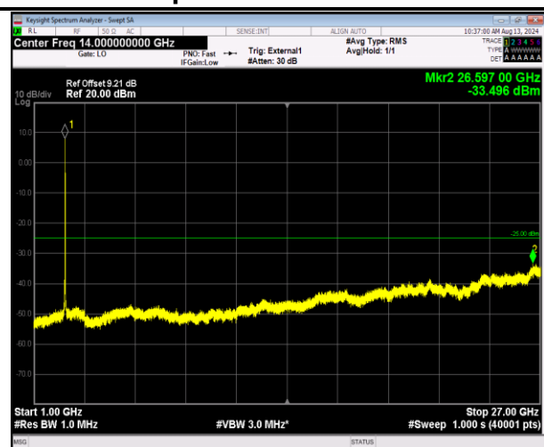
41-41-20MHz-5MHz-QPSK-QPSK-40715-40832-100RB# 0-25RB#0-1000~27000MHz-PASS
