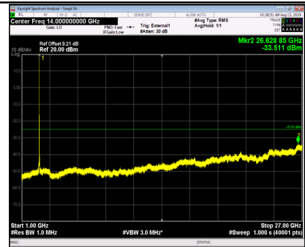
41-41-20MHz-5MHz-QPSK-QPSK-41090-41207-1RB#0-ORB#0-1000~27000MHz-PASS
