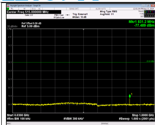
41-41-20MHz-20MHz-QPSK-QPSK-40641-40839-1RB# 0-ORB#0-30~1000MHz-PASS
