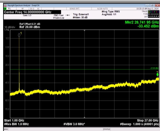
41-41-20MHz-5MHz-QPSK-QPSK-40715-40832-1RB#0-1RB#24-1000~27000MHz-PASS
