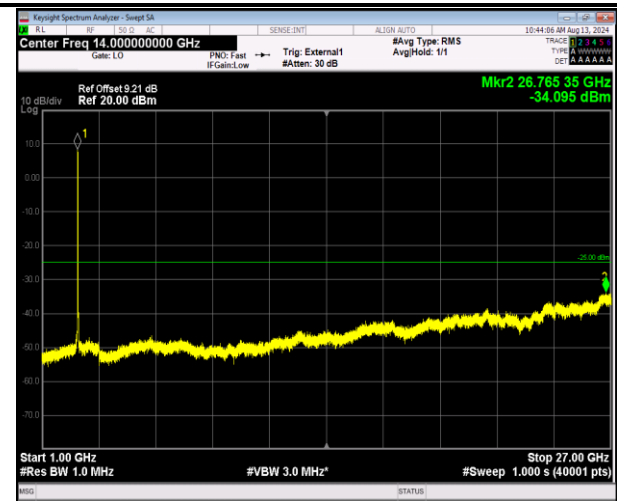
41-41-20MHz-5MHz-QPSK-QPSK-41090-41207-100RB# 0-25RB#0-1000~27000MHz-PASS
