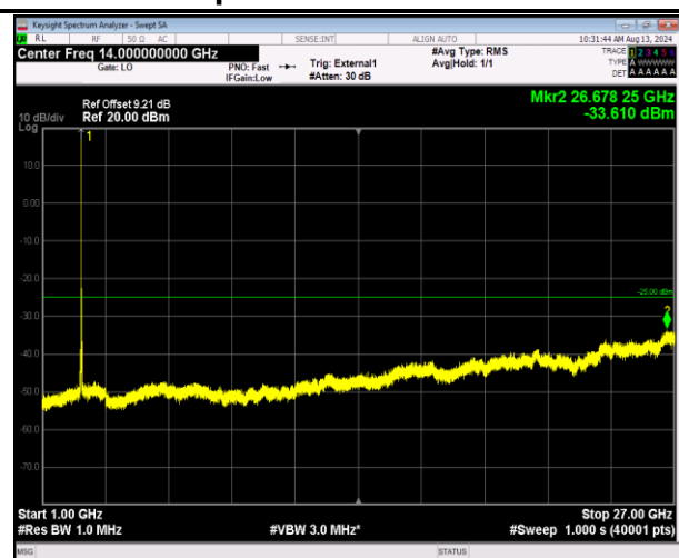
41-41-20MHz-5MHz-QPSK-QPSK-40715-40832-1RB#0-ORB#0-1000~27000MHz-PASS
