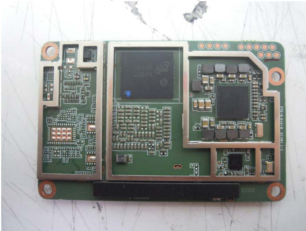
[WLAN,BT module Rear]
