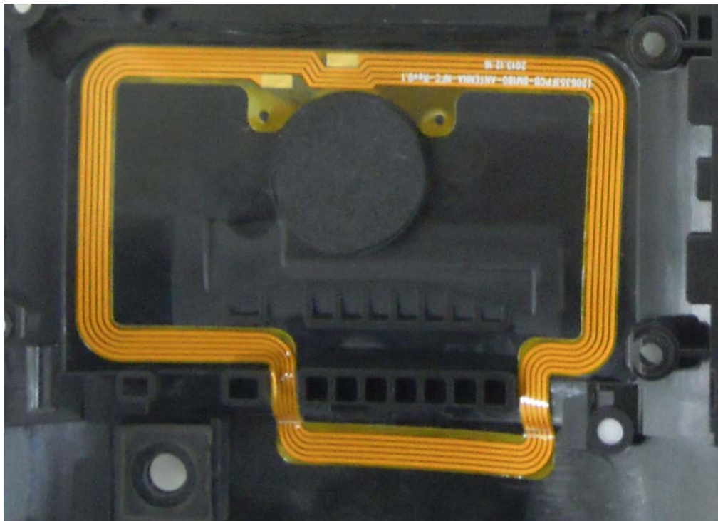
NFC Antenna
