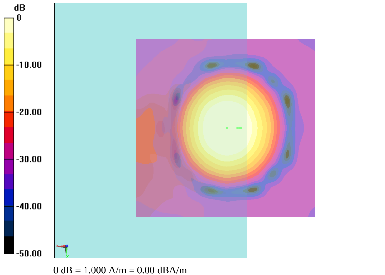
Fig B.12 T-Coil WCDMA 1900
