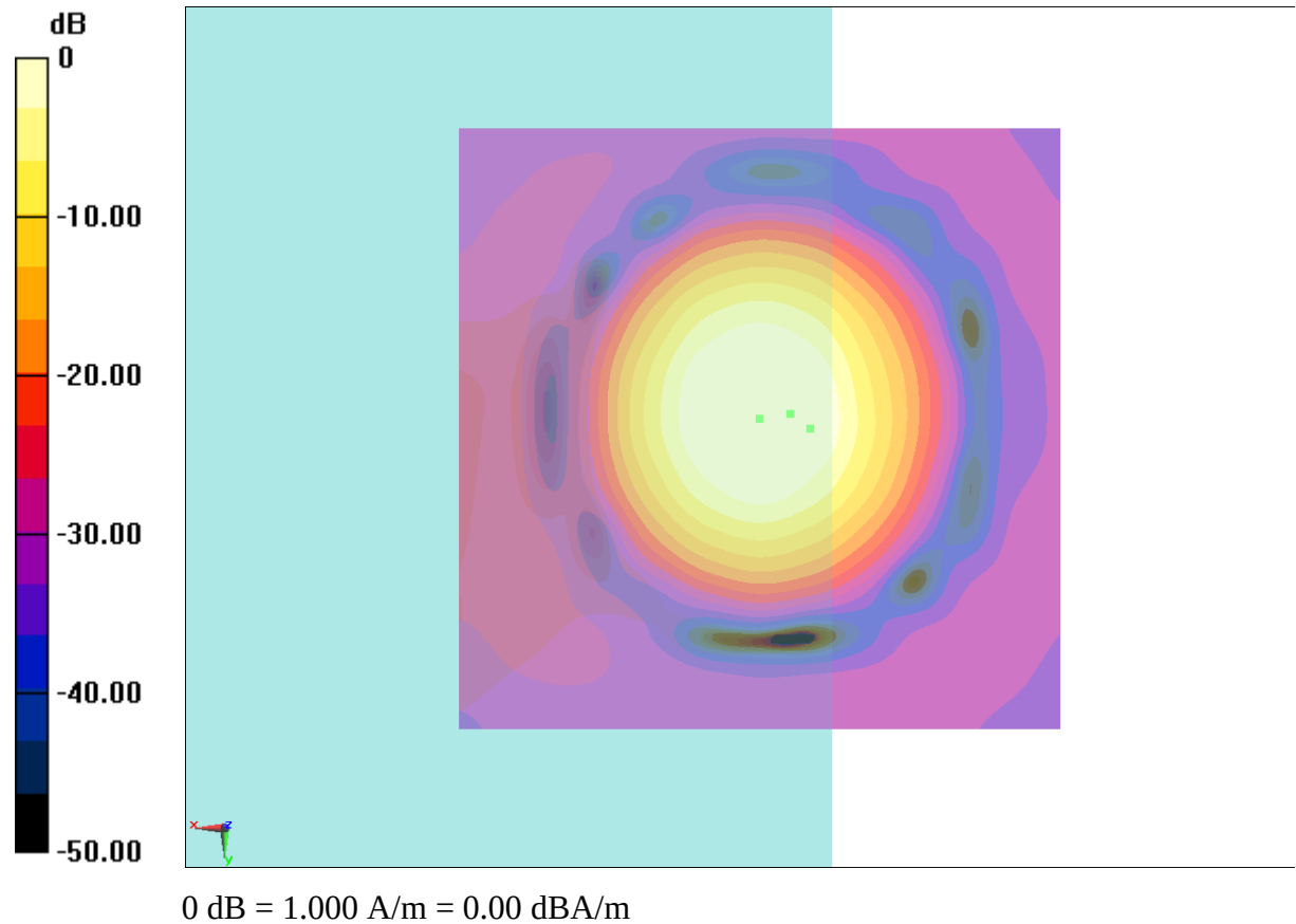
Fig B.9 T-Coil WCDMA 850
