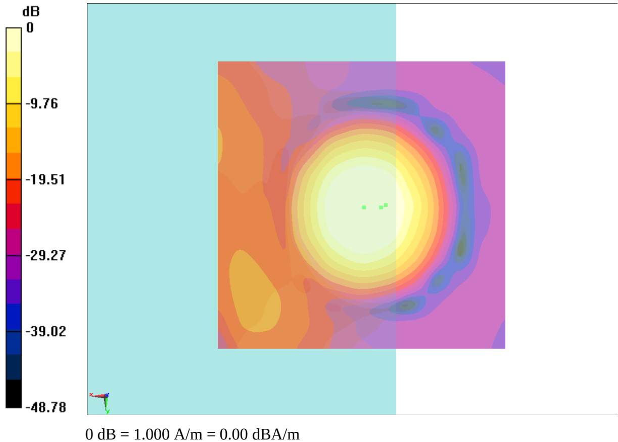
Fig B.3 T-Coil GSM 850
