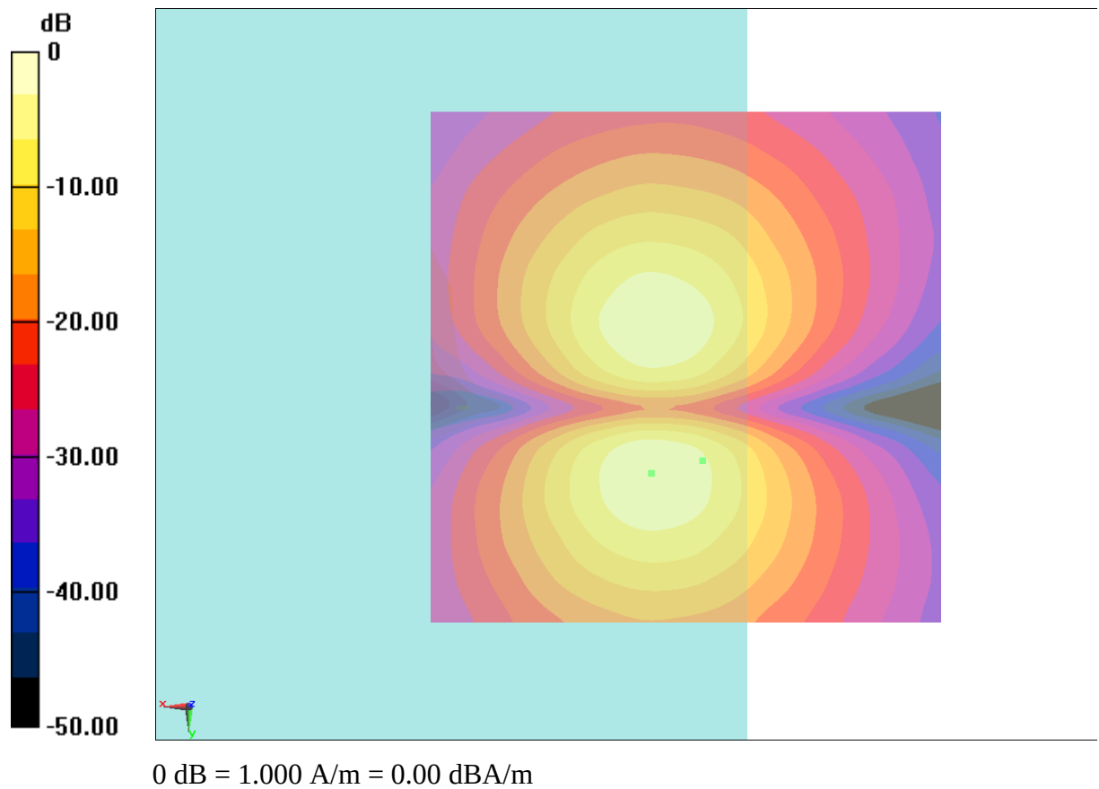
Fig B.11 T-Coil WCDMA 1900
