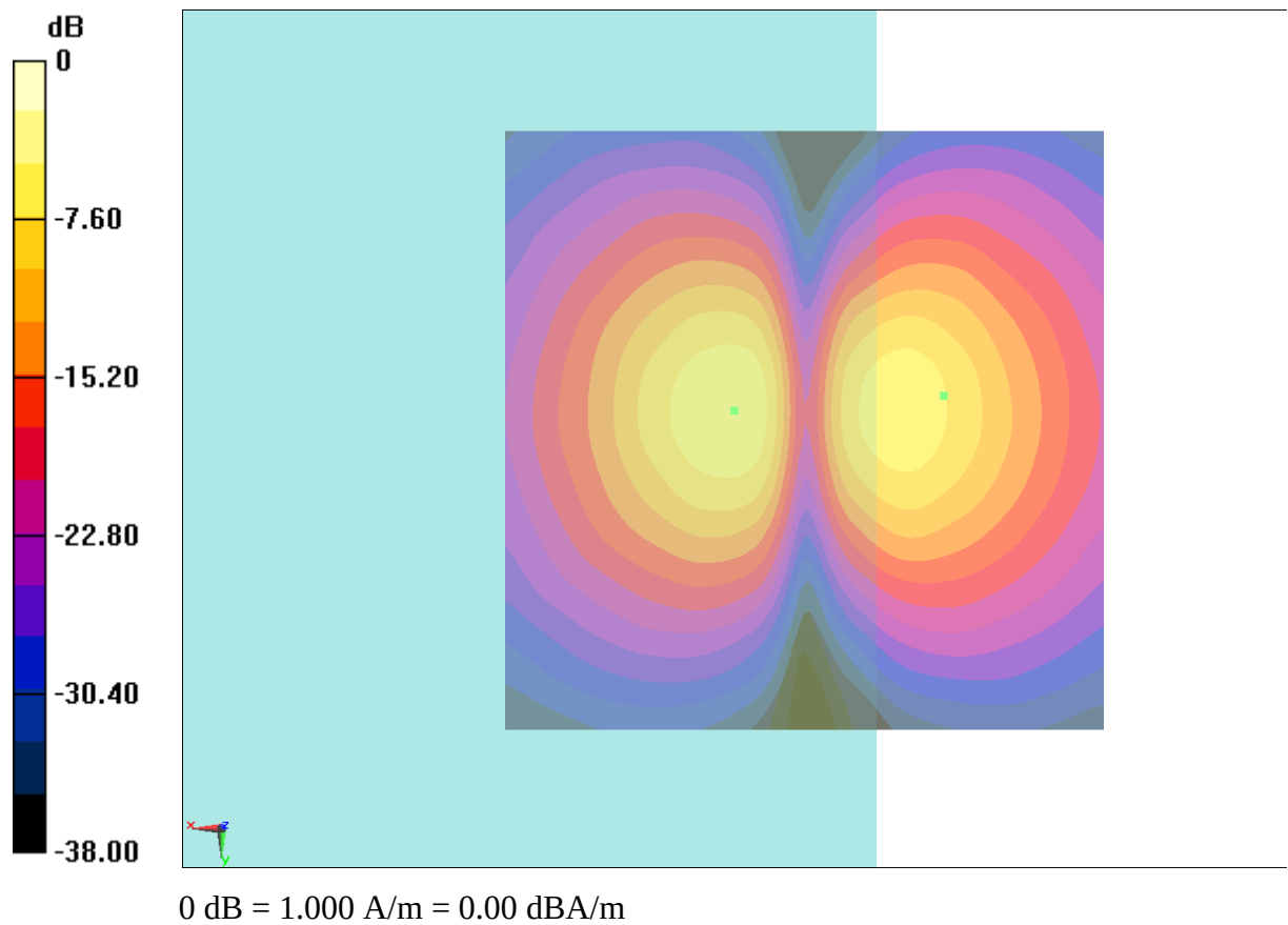
Fig B.7 T-Coil WCDMA 850
