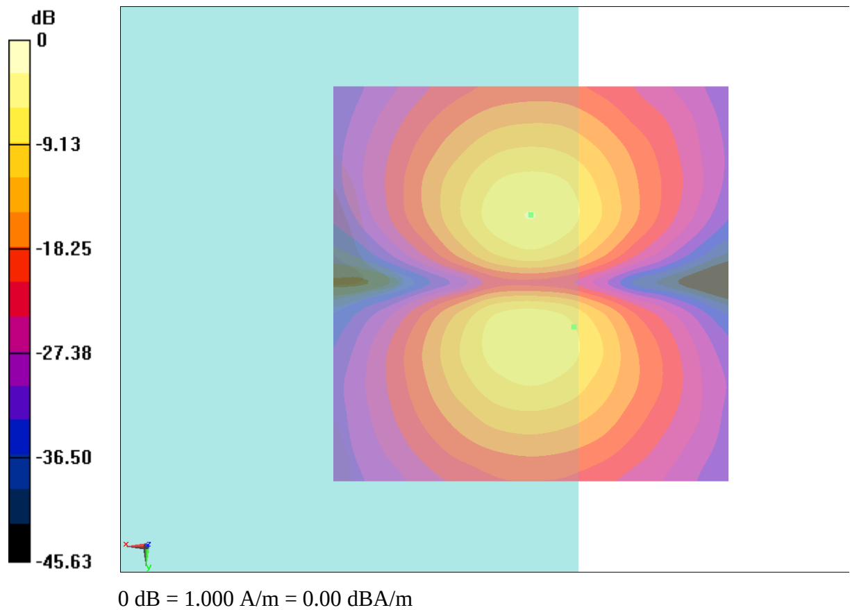
Fig B.8 T-Coil WCDMA 850
