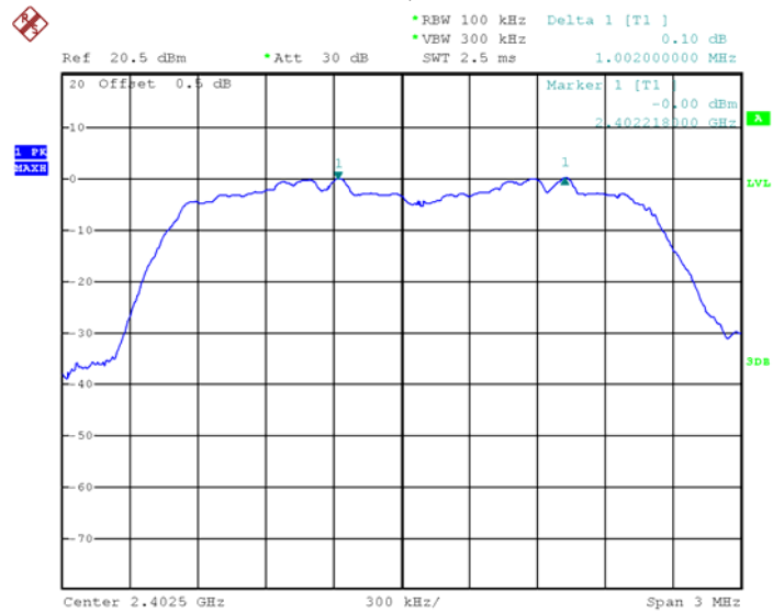
\pi/4 DQPSK Low Channel
