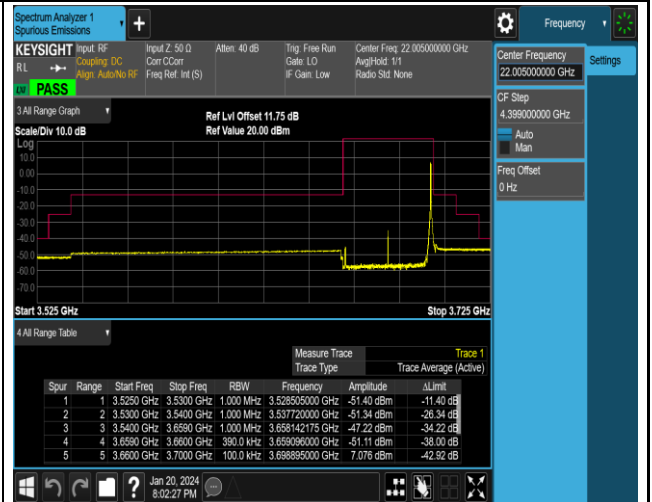
NTNV_N48_PC3_30_40_H_TID18_#1
