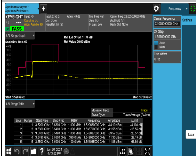
NTNV_N48_PC3_30_40_L_TID16_#1
