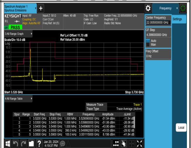
NTNV_N48_PC3_30_40_L_TID17_#1
