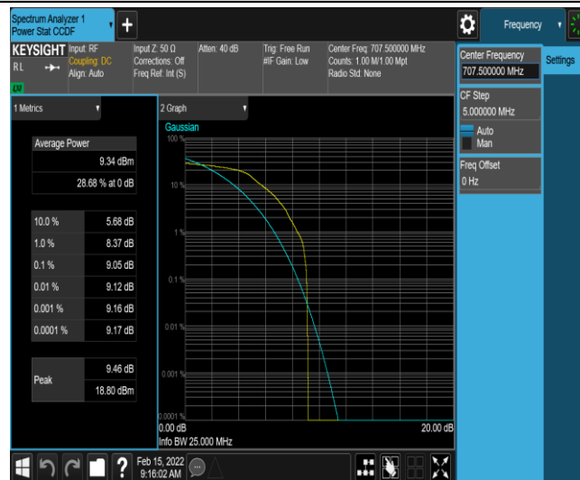
Band12-3MHz-QPSK-23095-1-0-Low-9.05-≤13-PASS
