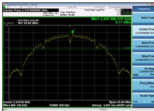
,Plot 1,Reference Level-802.11b ,2437MHz
