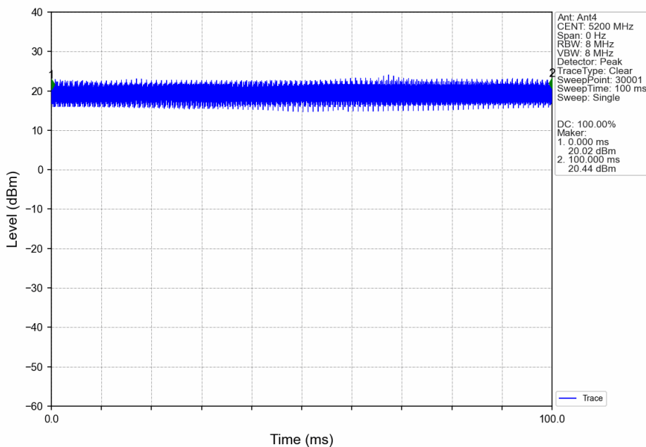
20M_MCH_5200MHz_Ant4_NTNV
