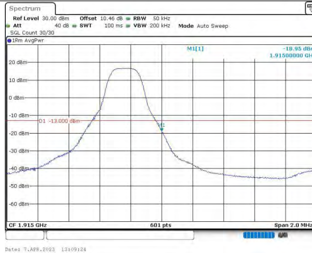
Band25-3MHz-QPSK-26675-1RB#14
