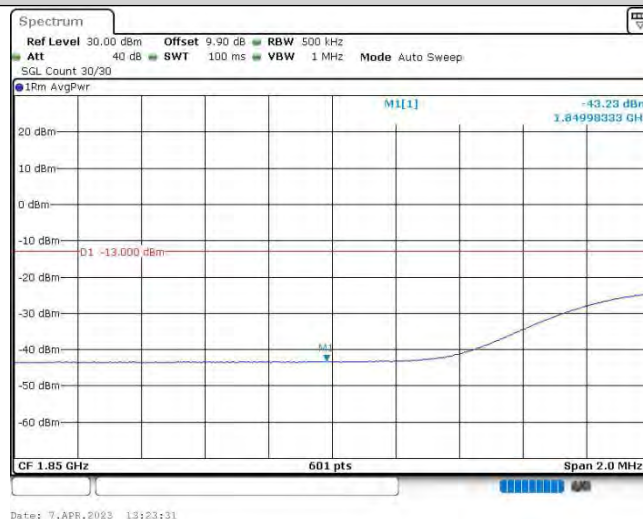
Band25-20MHz-QPSK-26140-1RB#99
