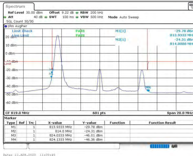
Band26@90-10MHz-QPSK-26740-1RB#0
