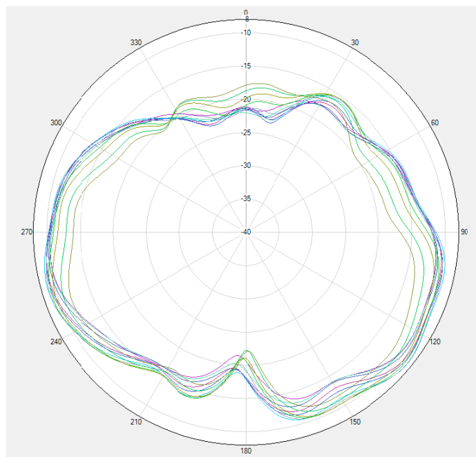
LTEB28 Phi=0deg
