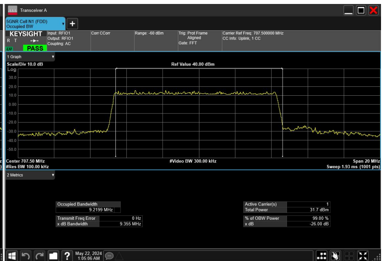
10MHz_15kHz_707.5MHz_DFT-s-OFDM 64 QAM_RB50@0
