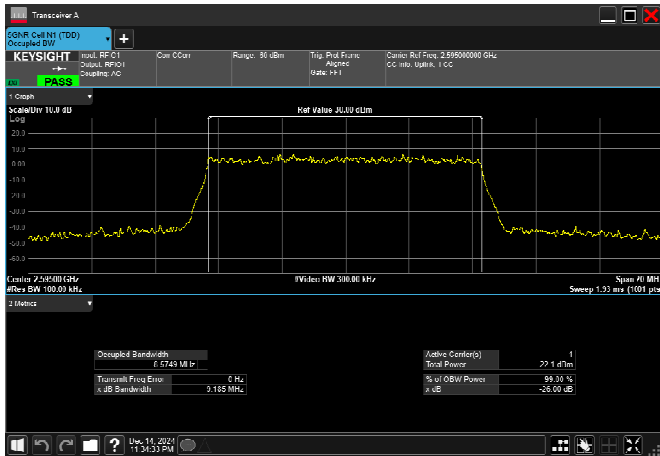
n38_10MHz_30kHz_2595MHz_CP-OFDM 256 QAM_RB24@0
