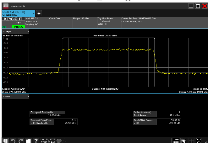
n38_25MHz_30kHz_2595MHz_DFT-s-OFDM QPSK_RB64@0
