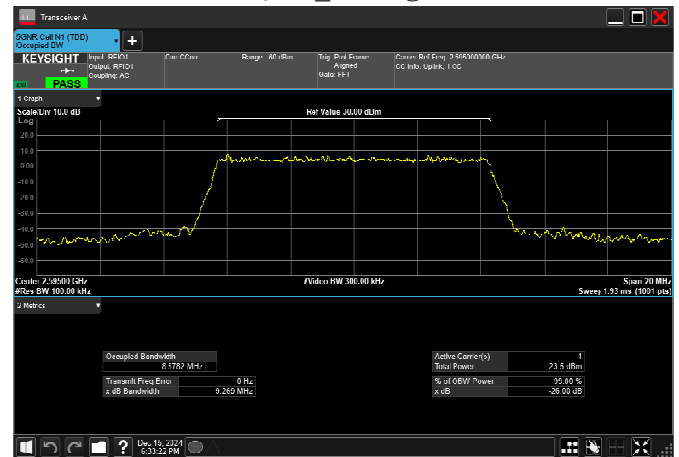
n38_10MHz_30kHz_2595MHz_CP-OFDM QPSK_RB24@0
