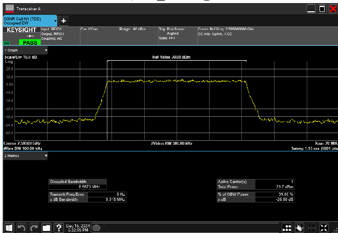
n38_10MHz_30kHz_2595MHz_DFT-s-OFDM 256 QAM_RB24@0
