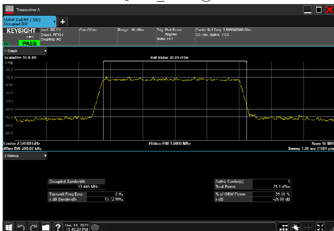
n38_15MHz_30kHz_2595MHz_DFT-s-OFDM QPSK_RB36@0
