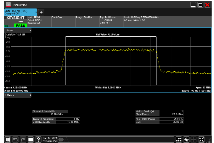
n38_25MHz_30kHz_2595MHz_DFT-s-OFDM \pi/2 BPSK_RB64@0
