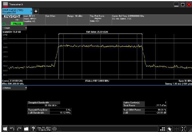
n38_20MHz_30kHz_2595MHz_CP-OFDM 256 QAM_RB51@0
