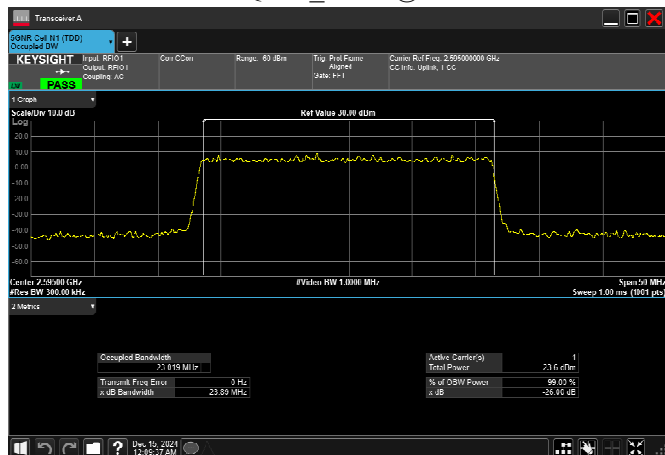
n38_25MHz_30kHz_2595MHz_CP-OFDM QPSK_RB65@0
