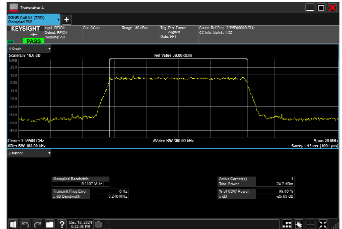
n38_10MHz_30kHz_2595MHz_DFT-s-OFDM 64 QAM_RB24@0
