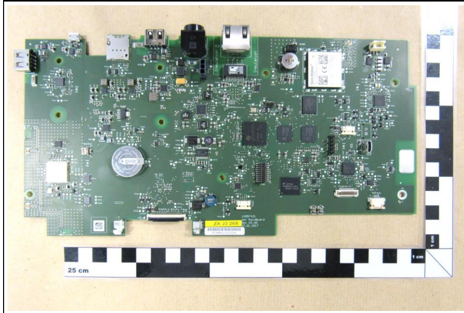
PCB Top
