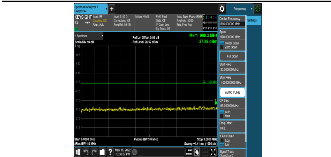
Band2-20MHz-16QAM-18700-1RB#0-Range3:30~1000MHz
