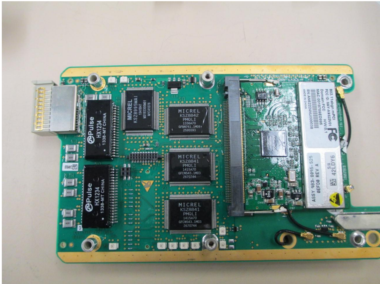
802Com_board_top
