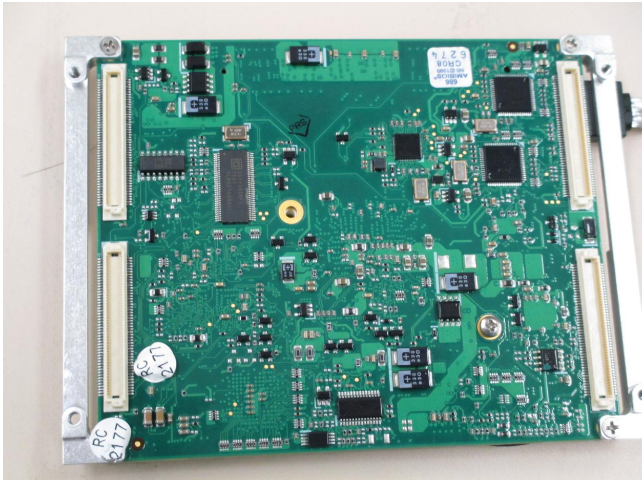
SBC_bottom
