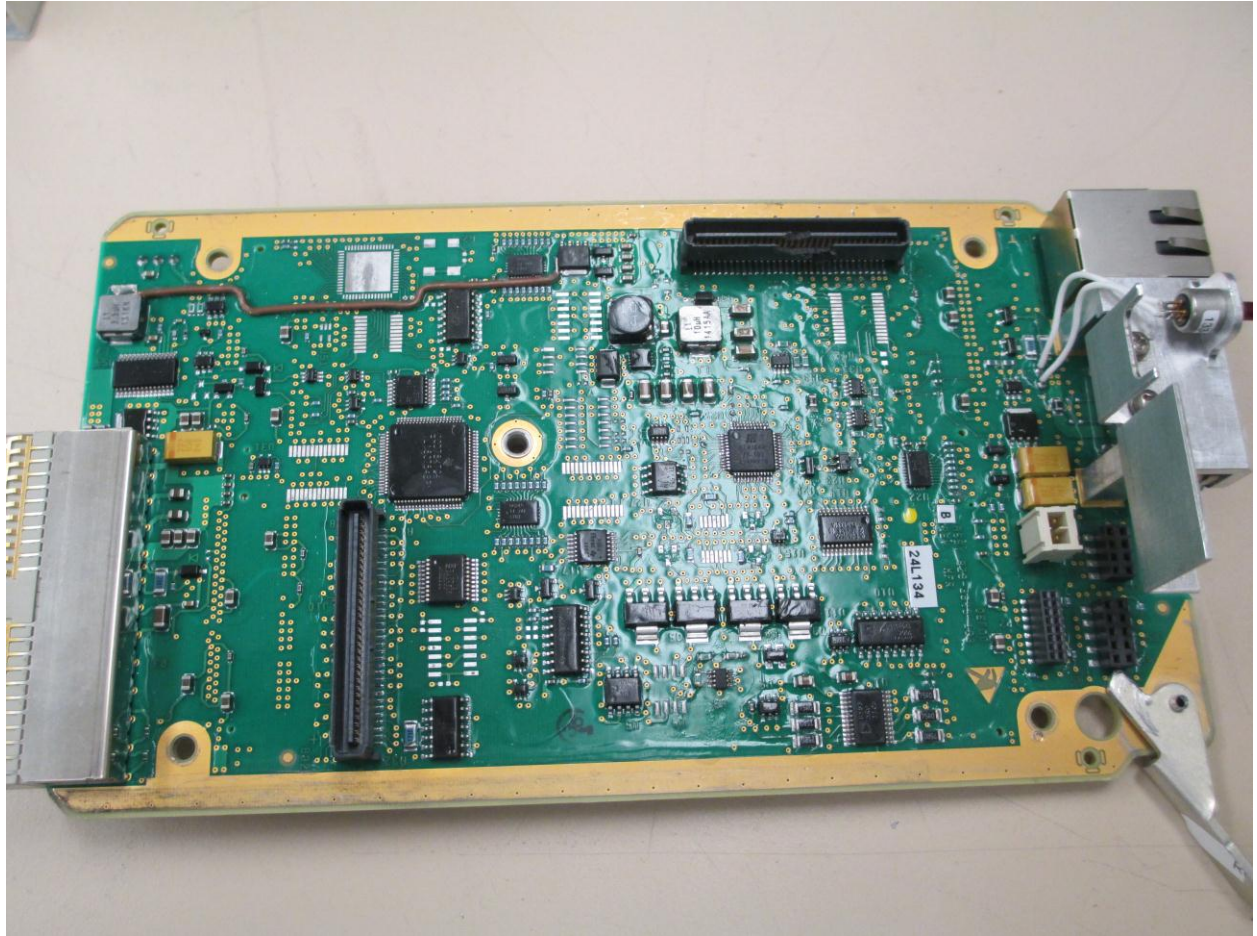
PC_Base_card_top
