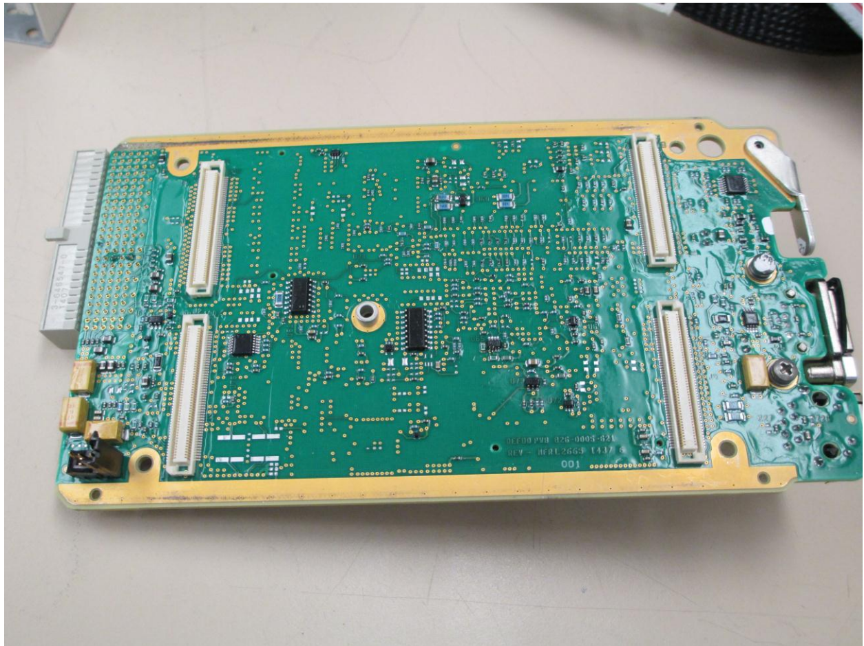
PC_Base_bottom
