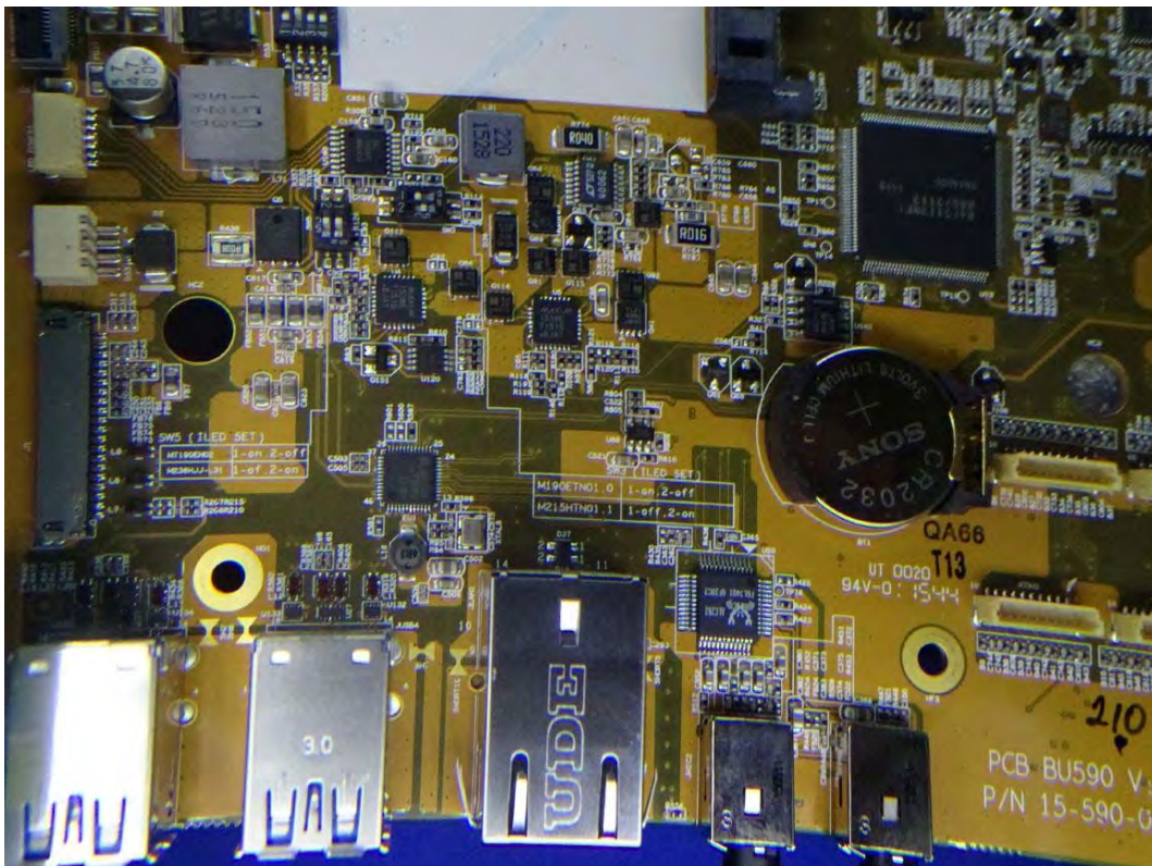
(104) EUT Photo
