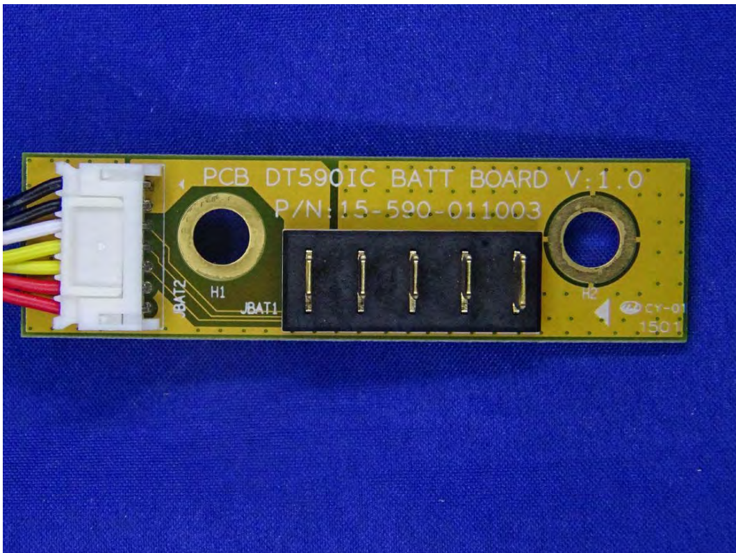
(114) EUT Photo
