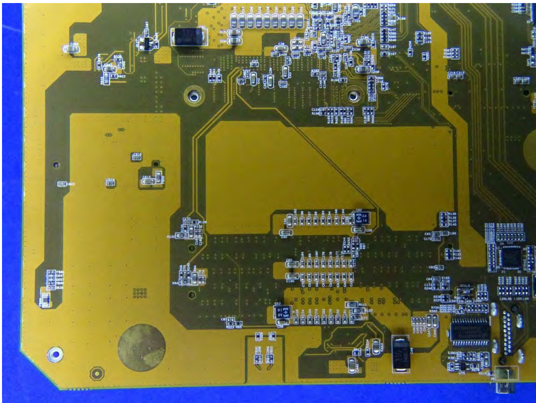
(110) EUT Photo
