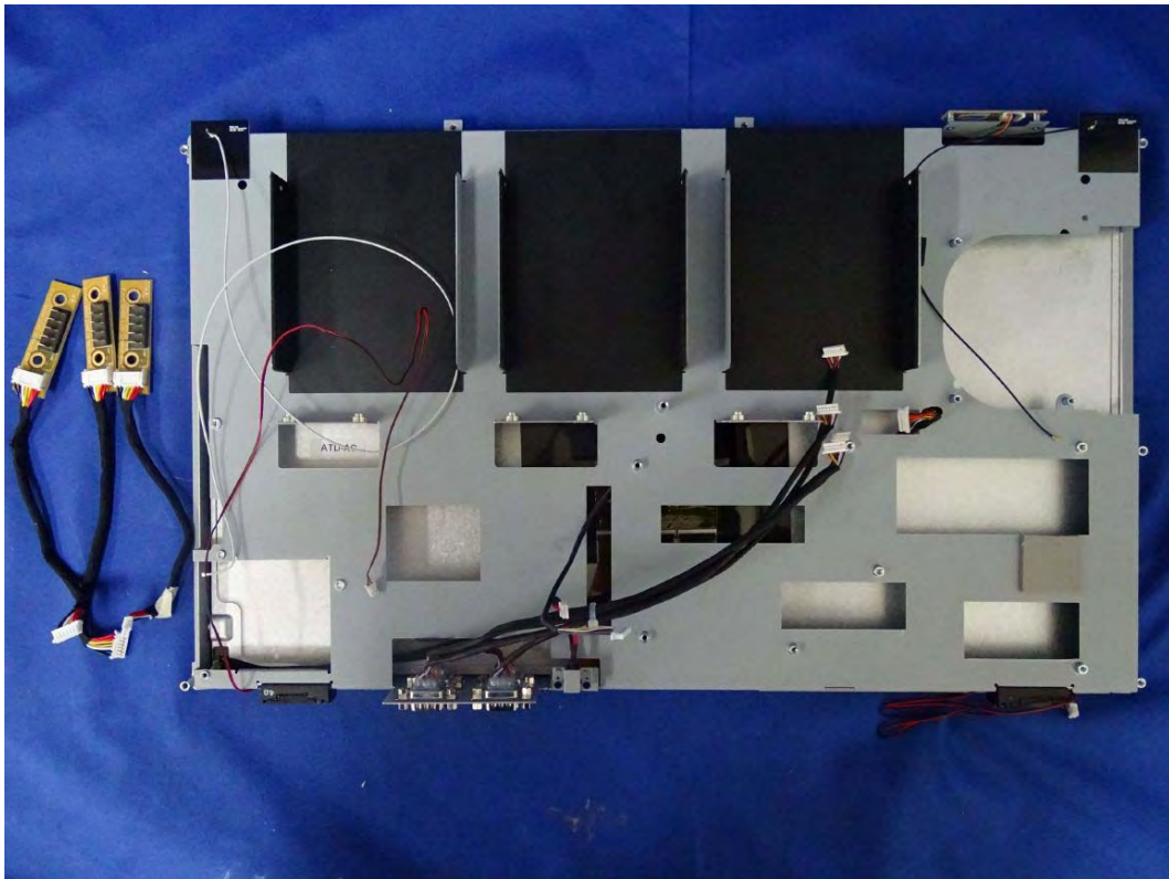
(113) EUT Photo
