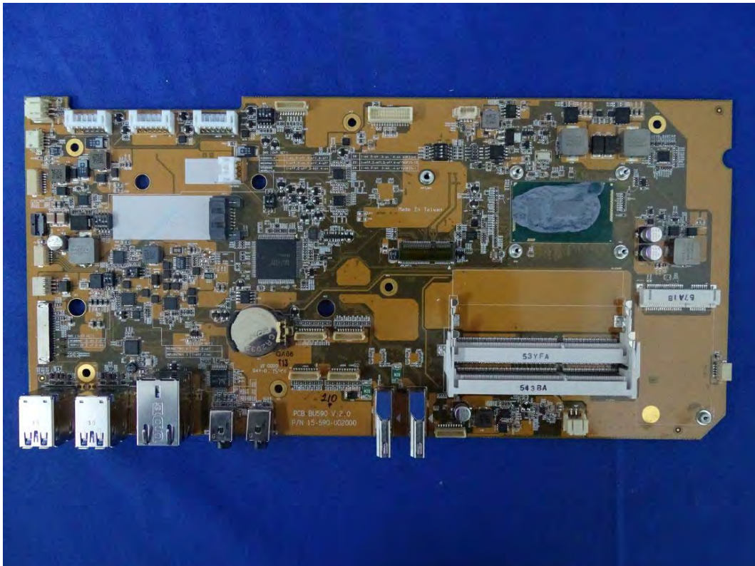
(102) EUT Photo
