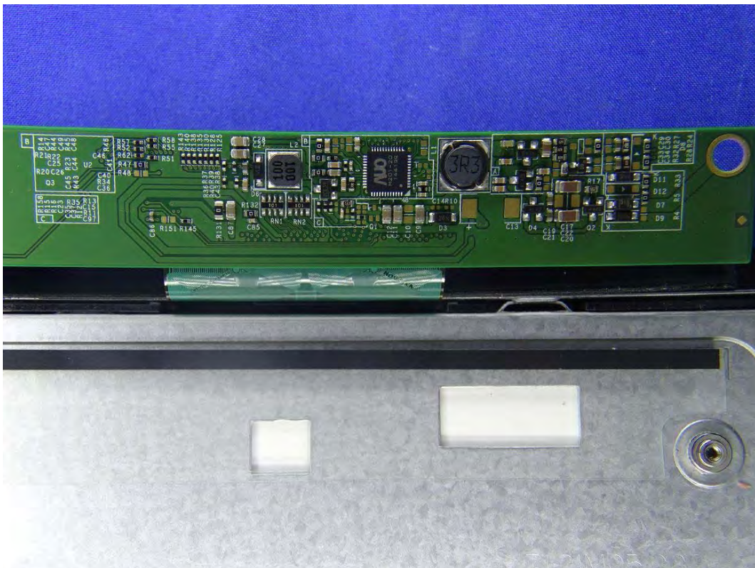
(130) EUT Photo
