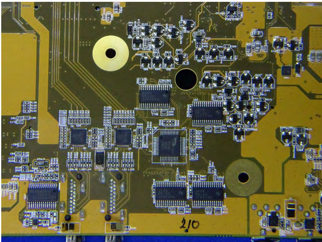
(112) EUT Photo
