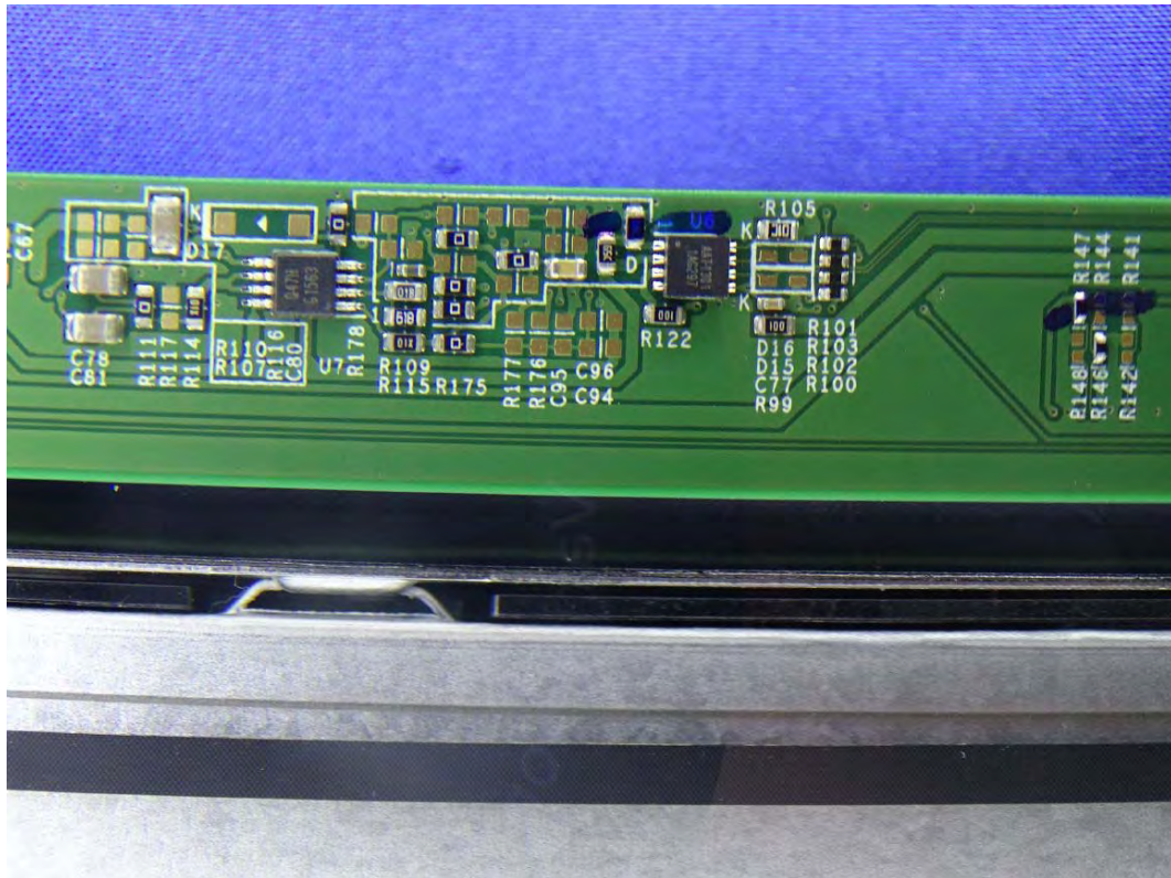
(127) EUT Photo
