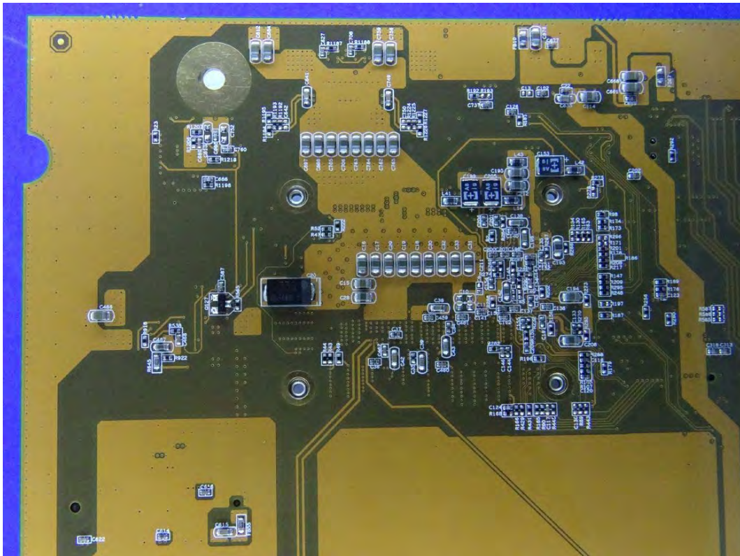
(109) EUT Photo
