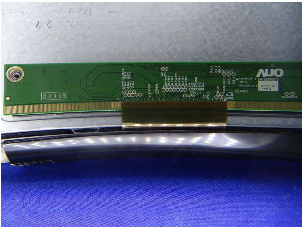
(132) EUT Photo
