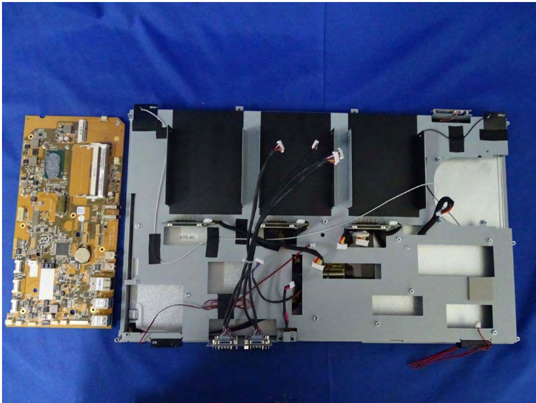
(101) EUT Photo
